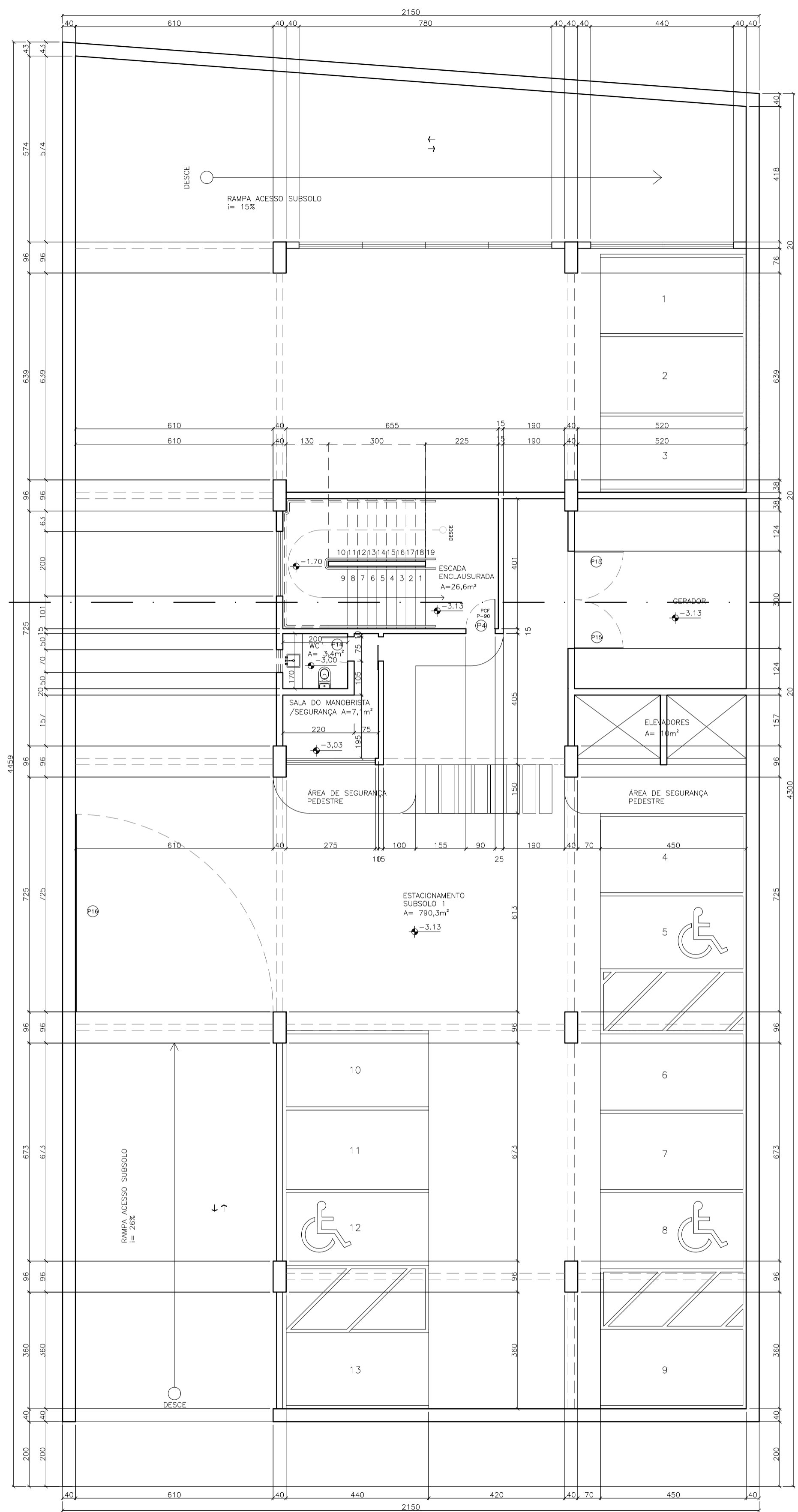
PLANTA TÉCNICA SUBSOLO 1 esc. 1:100
