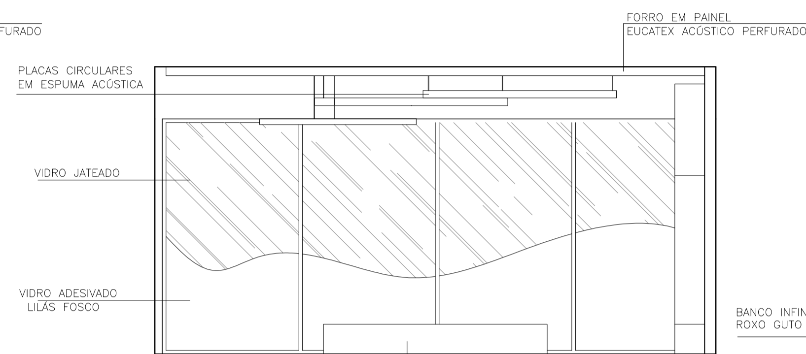
VISTA 02 SALA DE DESENHO E PINTURA ESCALA 1:50
