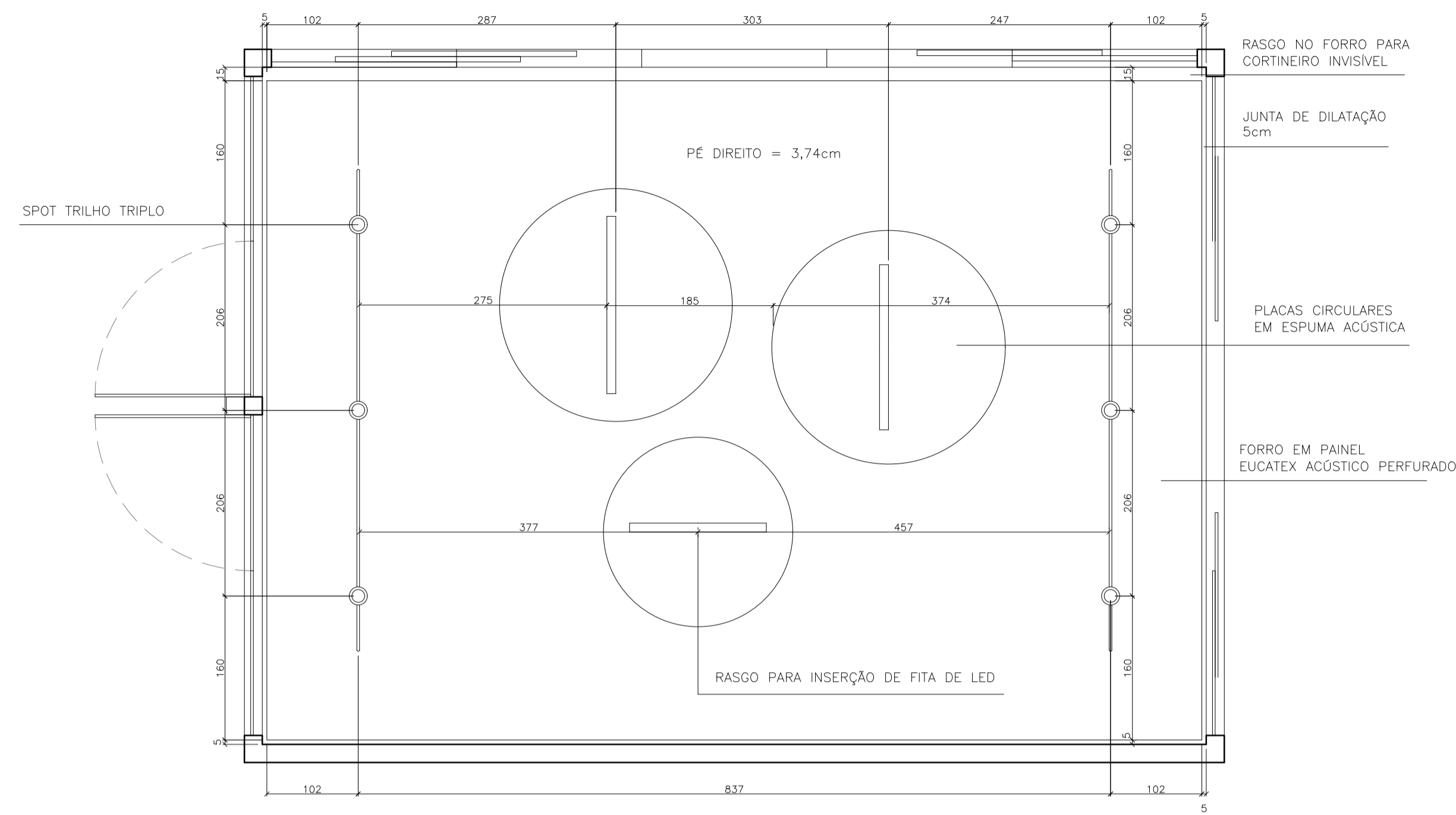
PLANTA DE FORRO SALA DE DESENHO E PINTURA ESCALA 1:50
