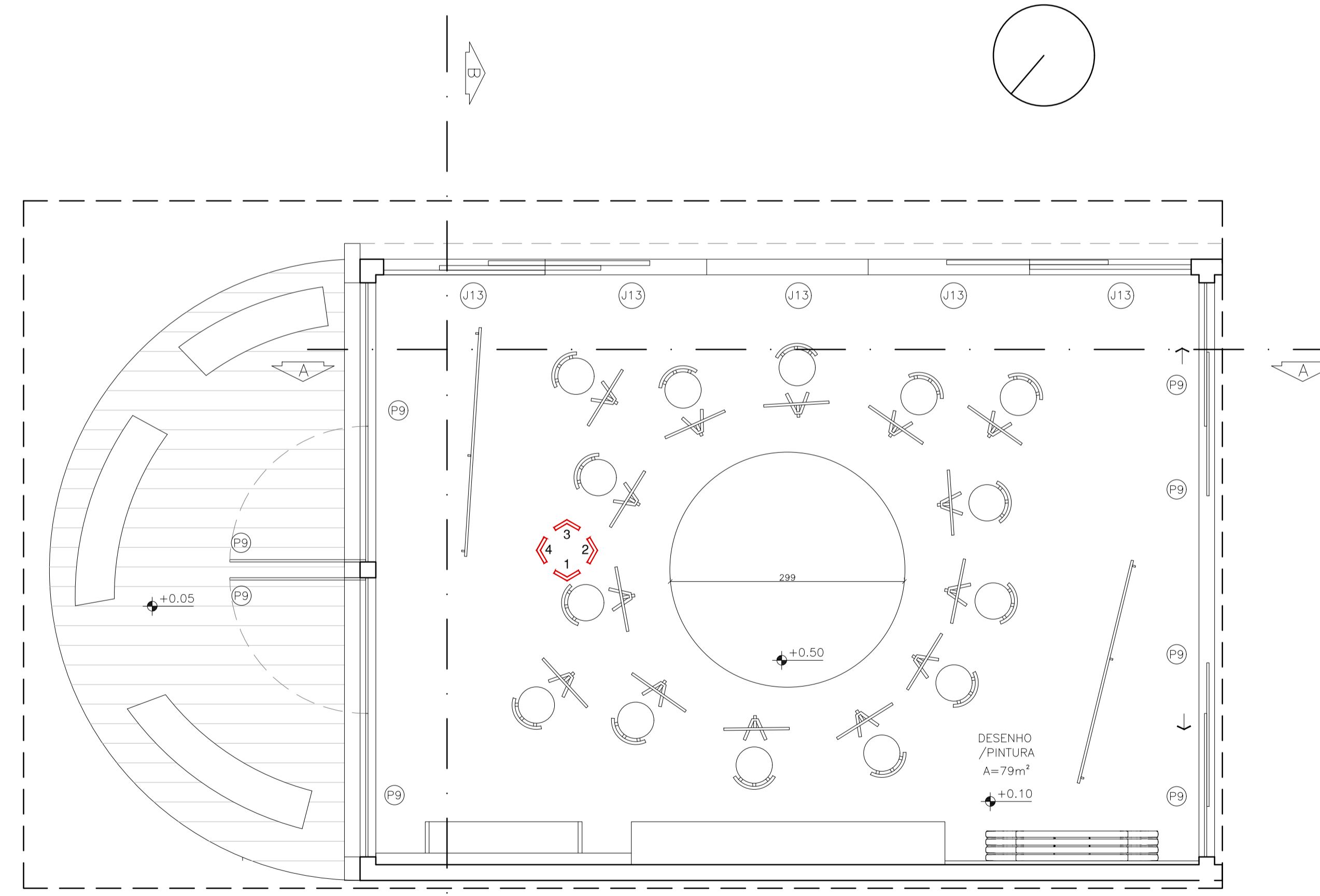
PLANTA LAYOUT – INTERIORES SALA DE DESENHO E PINTURA ESCALA 1:50
