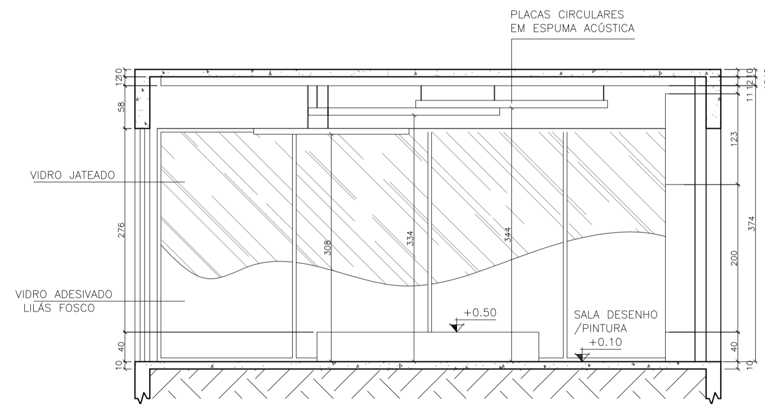
CORTE B SALA DE DESENHO E PINTURA ESCALA 1:50
