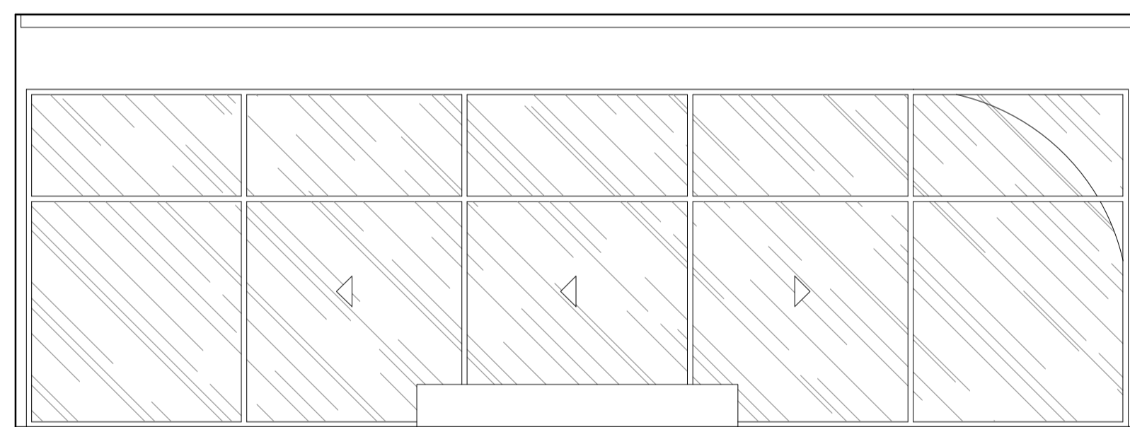
VISTA 03 SALA DE DESENHO E PINTURA ESCALA 1:50
