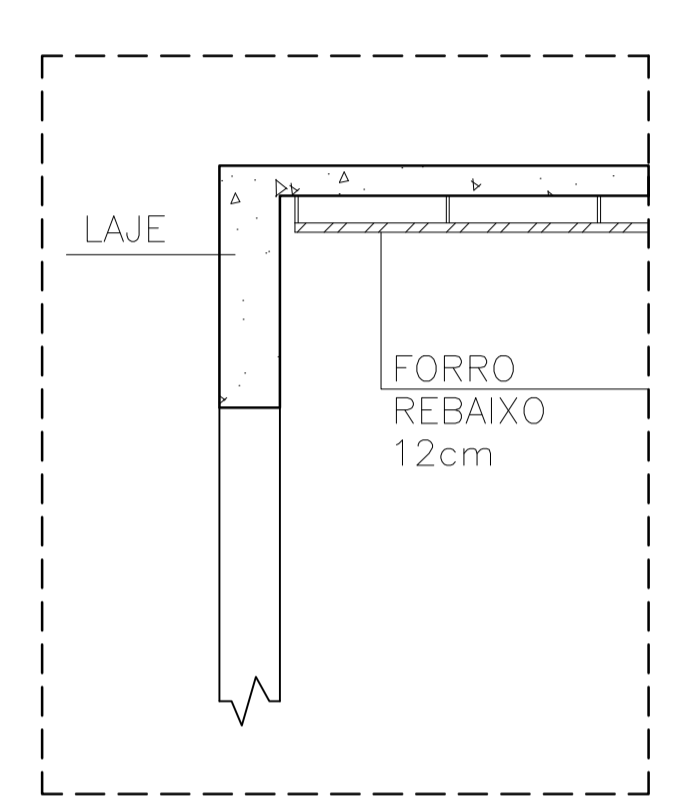
DETALHE FORRO ESCALA 1:25
