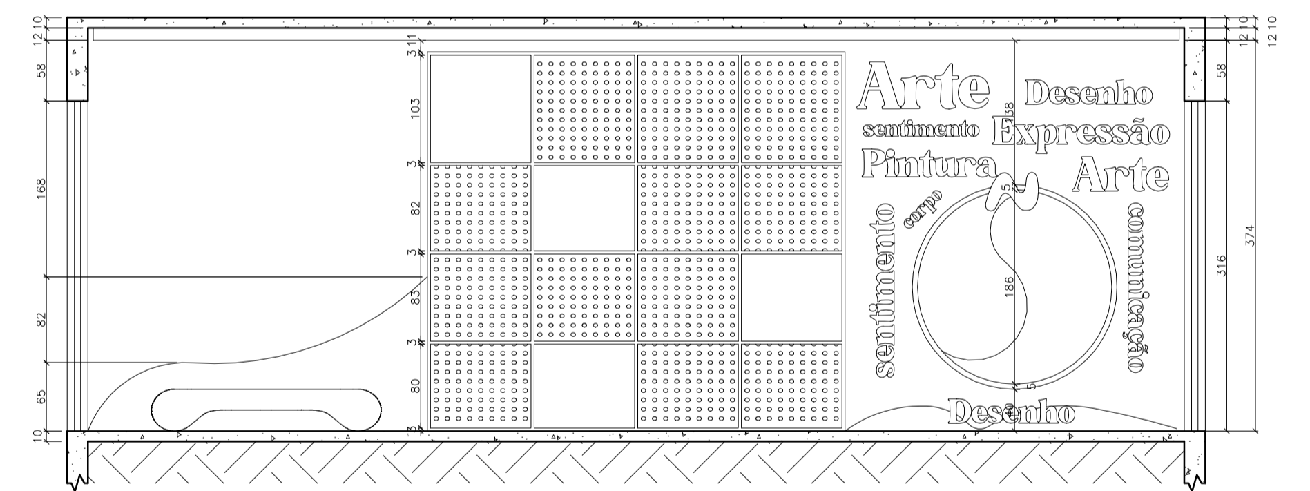
VISTA 01 SALA DE DESENHO E PINTURA ESCALA 1:50
