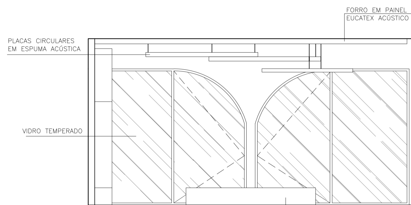
VISTA 04 SALA DE DESENHO E PINTURA ESCALA 1:50
