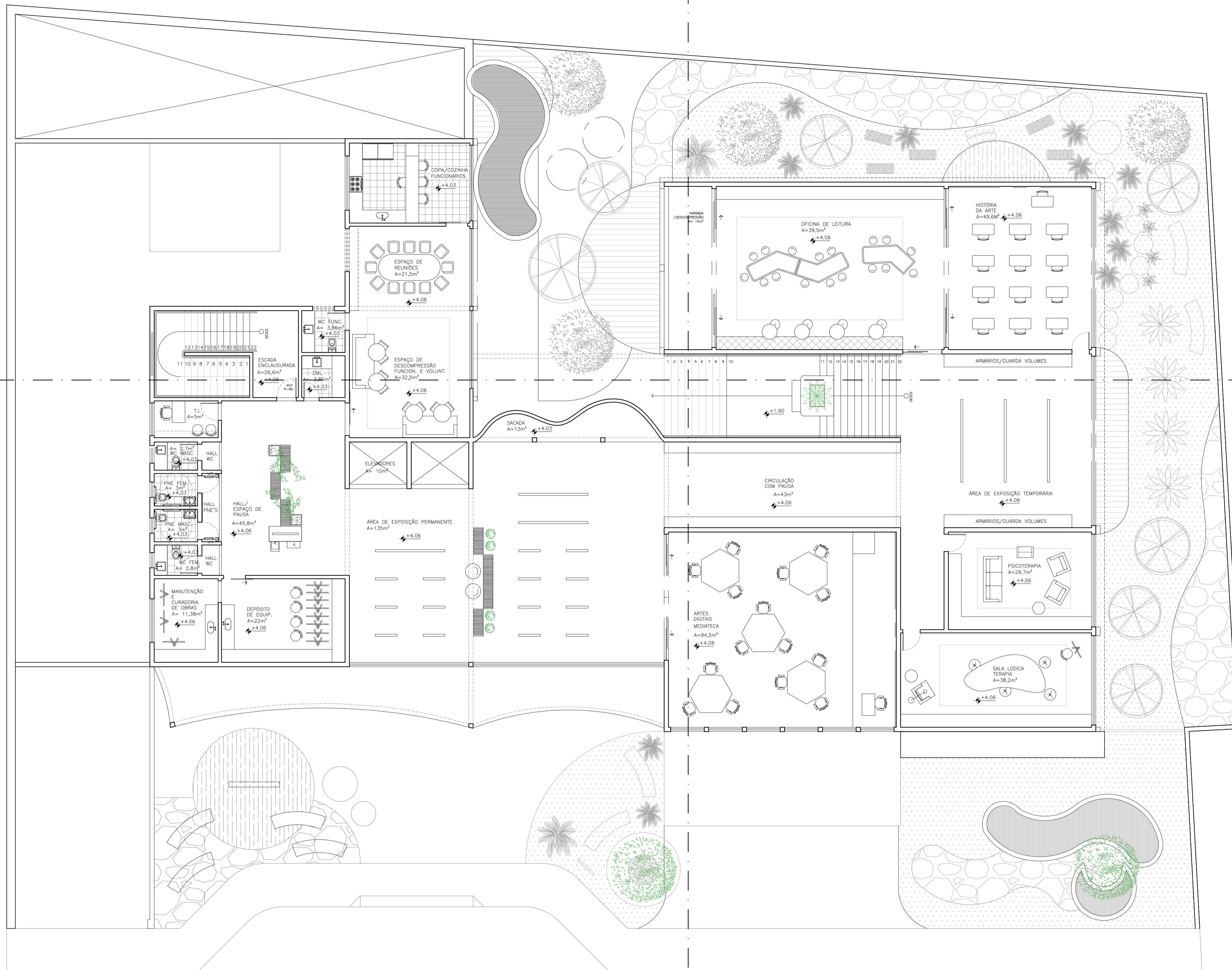
PLANTA LAYOUT 1 PAV. esc. 1:100
