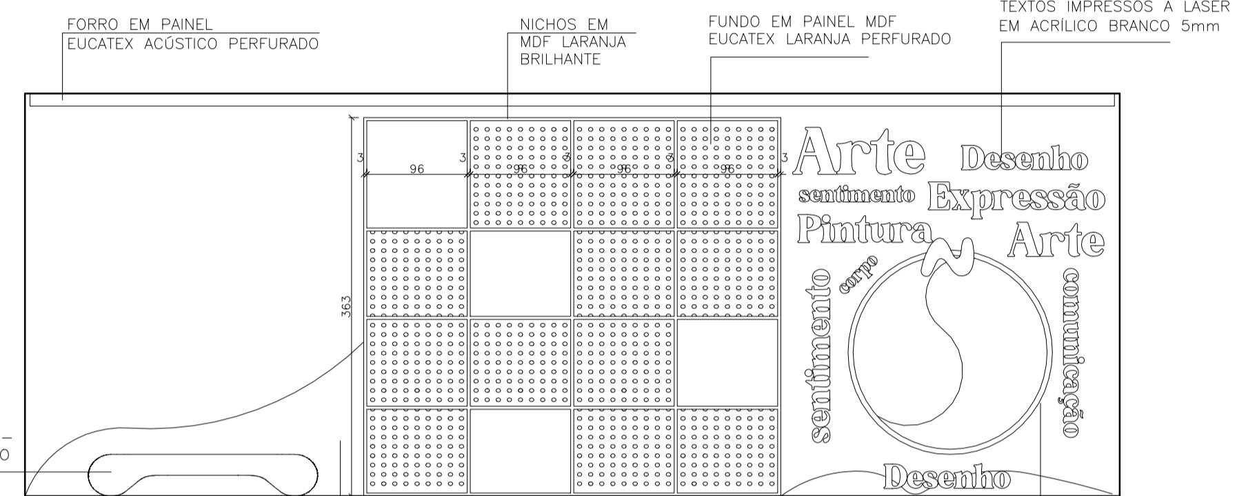
VISTA 01 SALA DE DESENHO E PINTURA ESCALA 1:50
