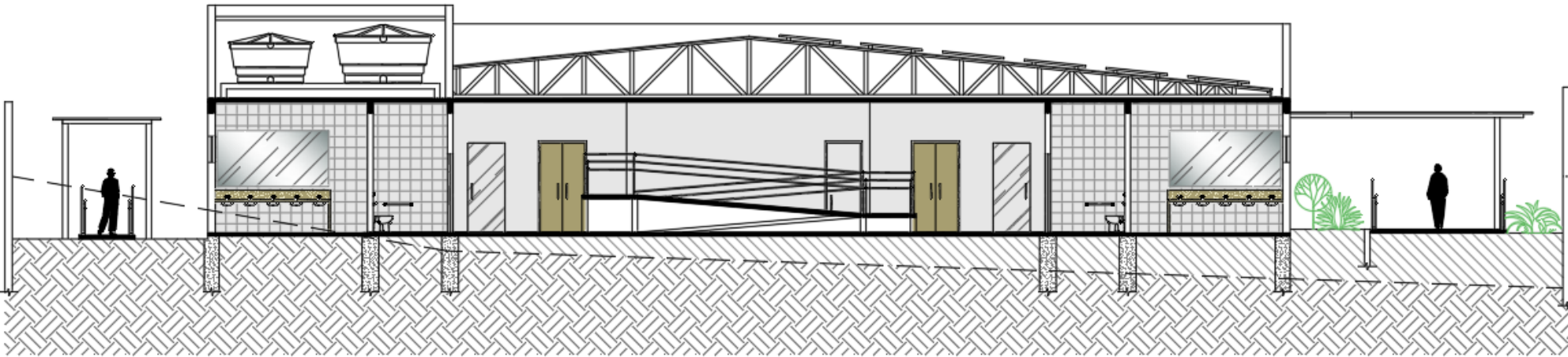
CORTE BB
