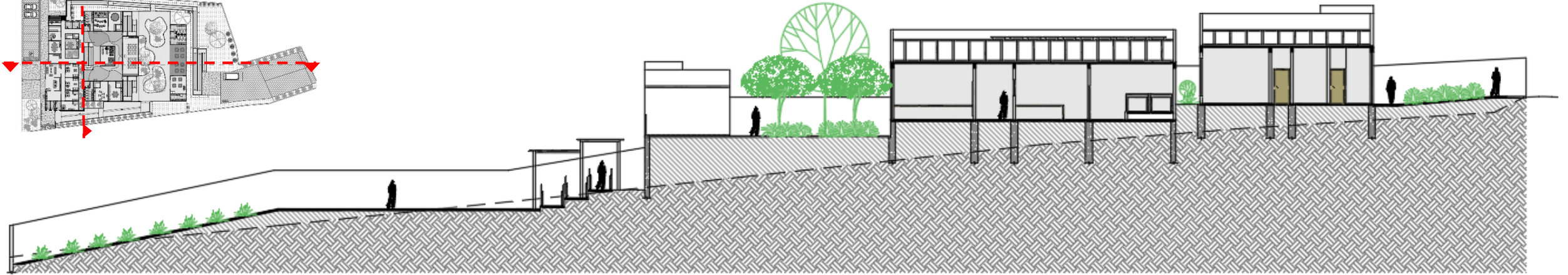
CORTE AA
