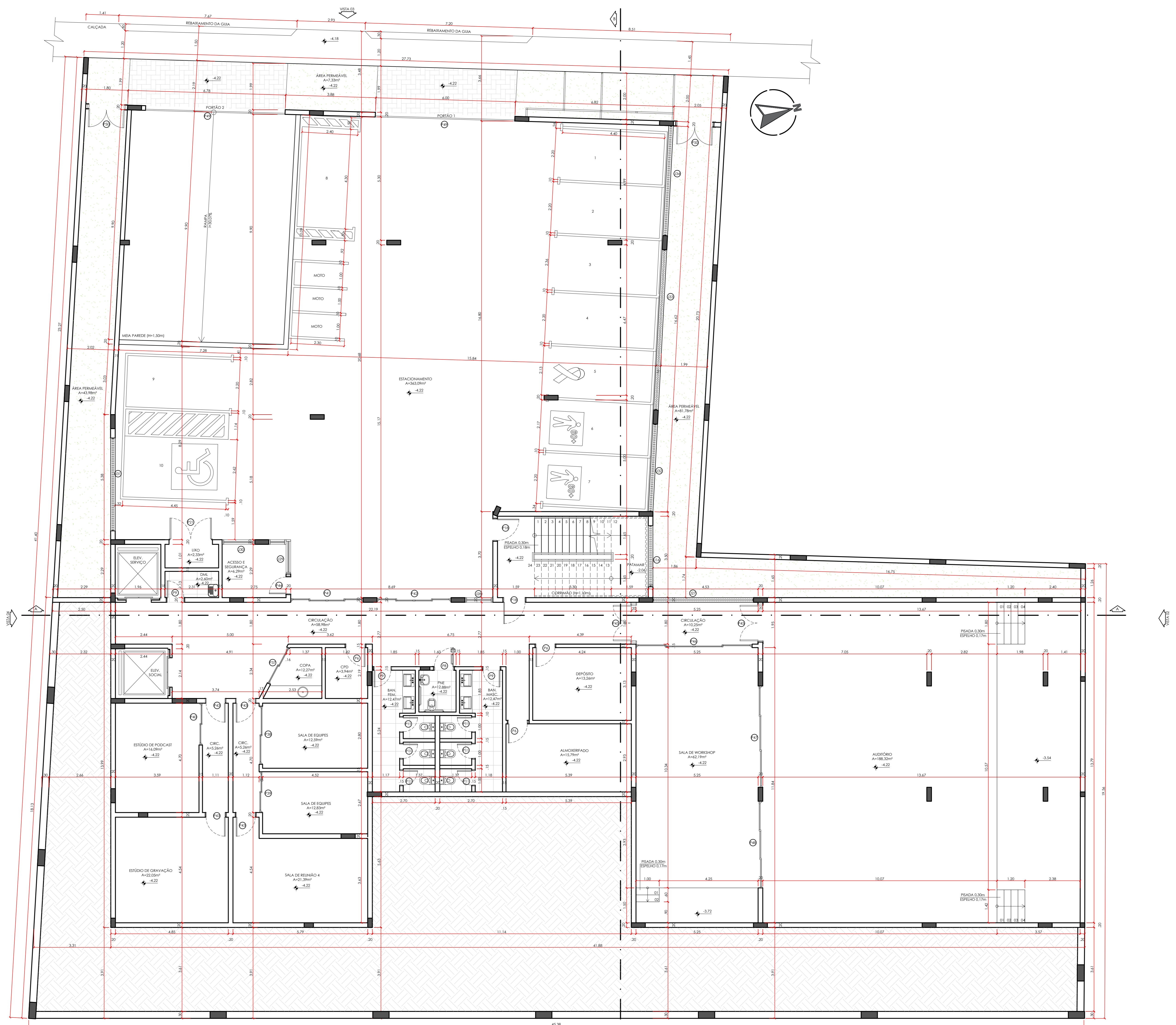
6 PLANTA BAIXA PAV. INFERIOR ±0=1.000,95m esc 1/75
