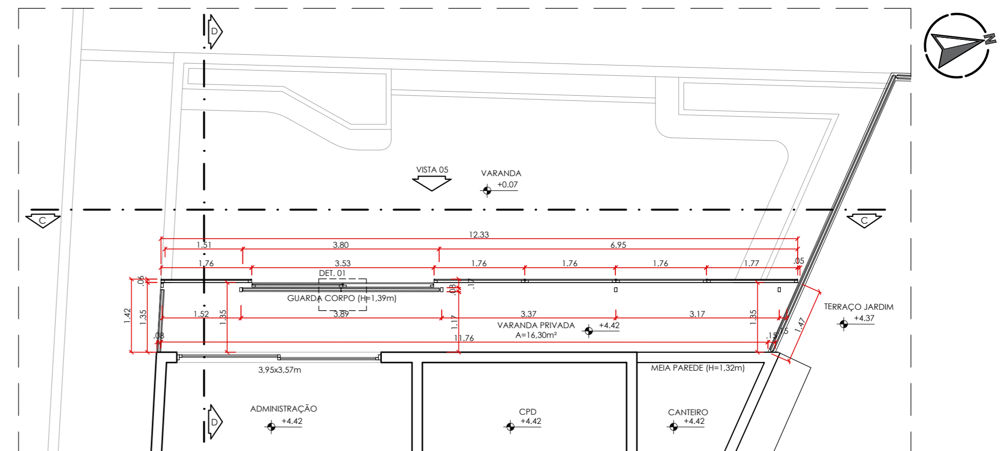
16 PLANTA BAIXA VARANDA 1º PAV. esc 1:75
