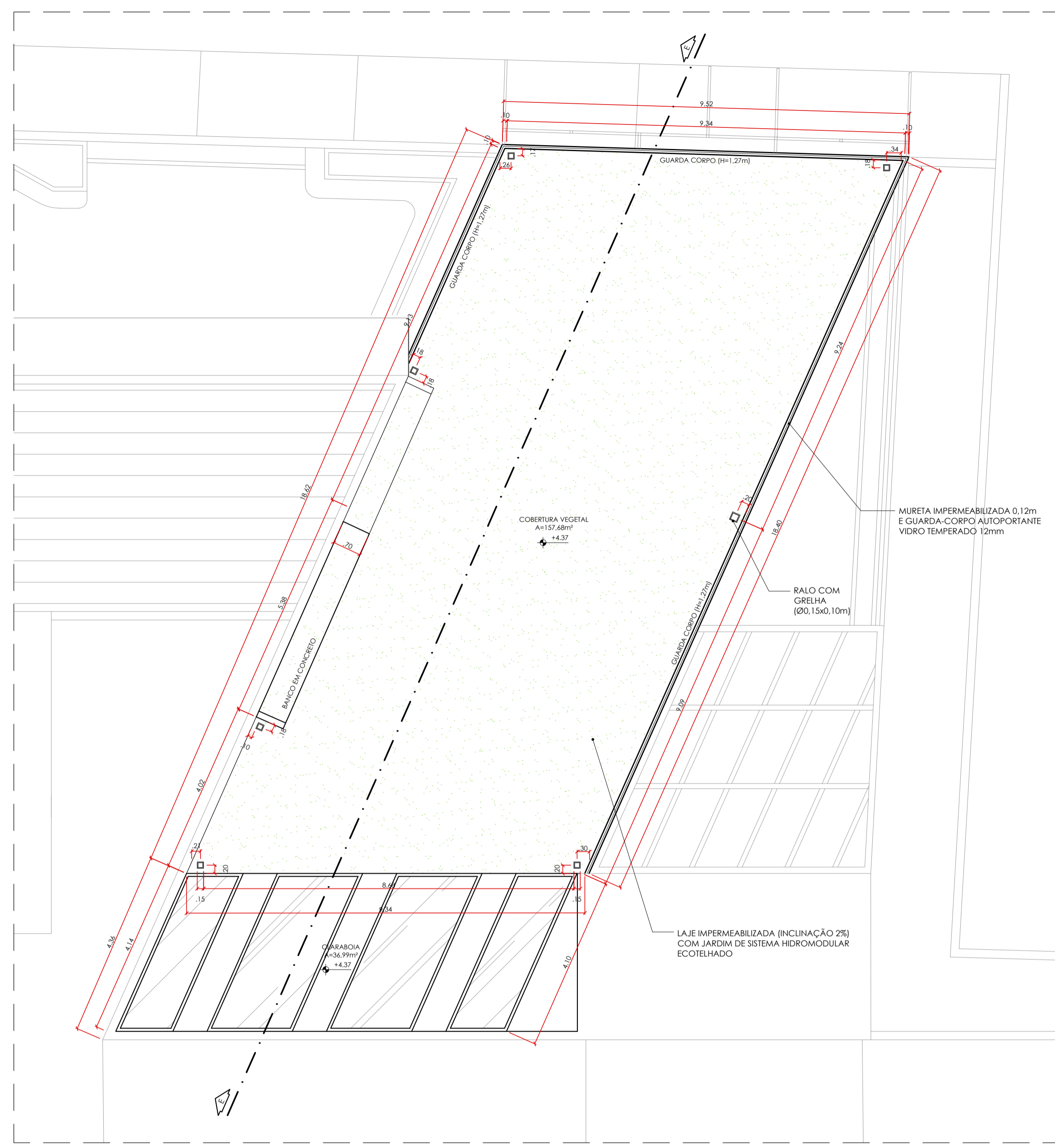
25 PLANTA COBERTURA TERRAÇO JARDIM esc 1:75
