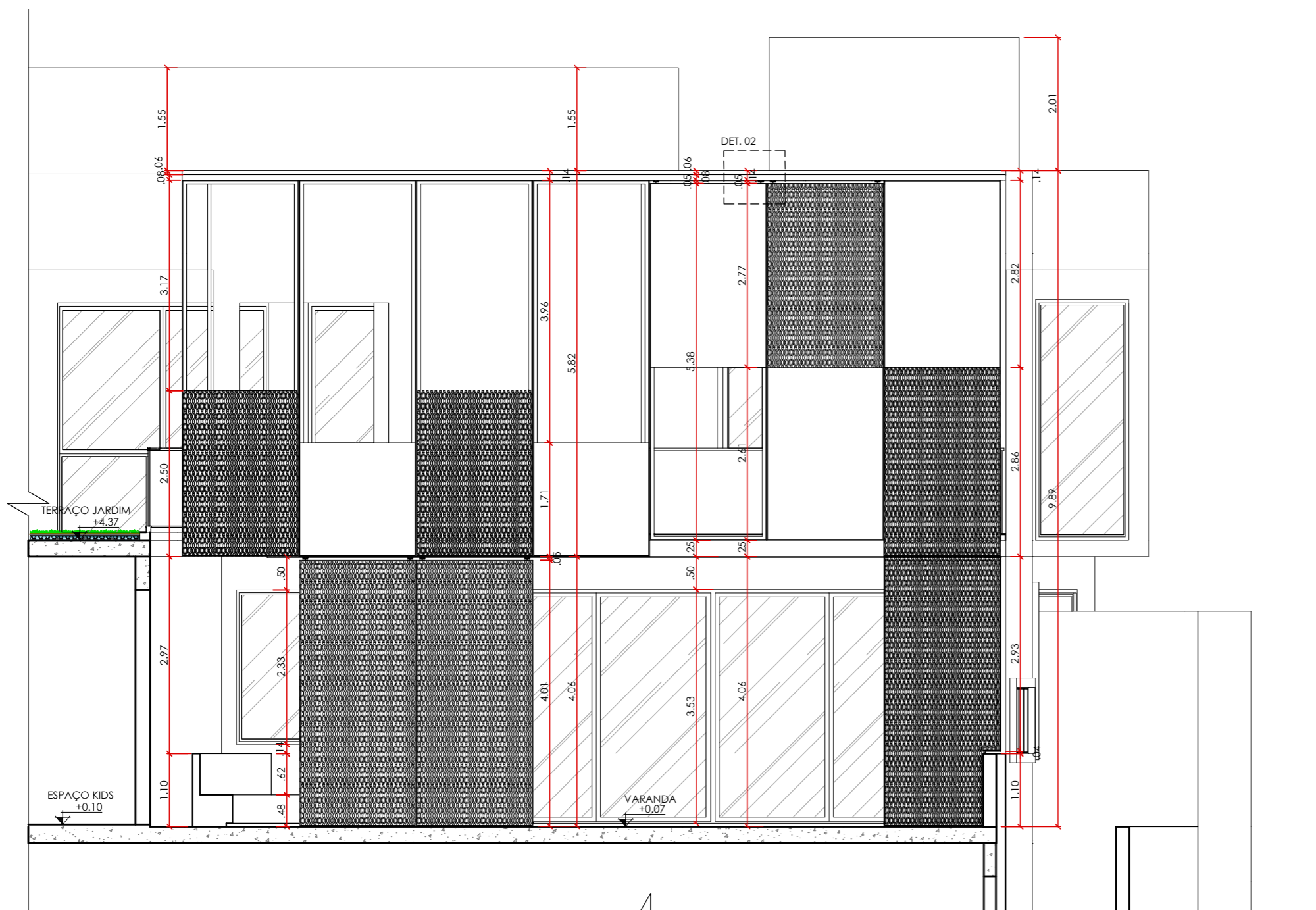
17 CORTE CC esc 1:75
