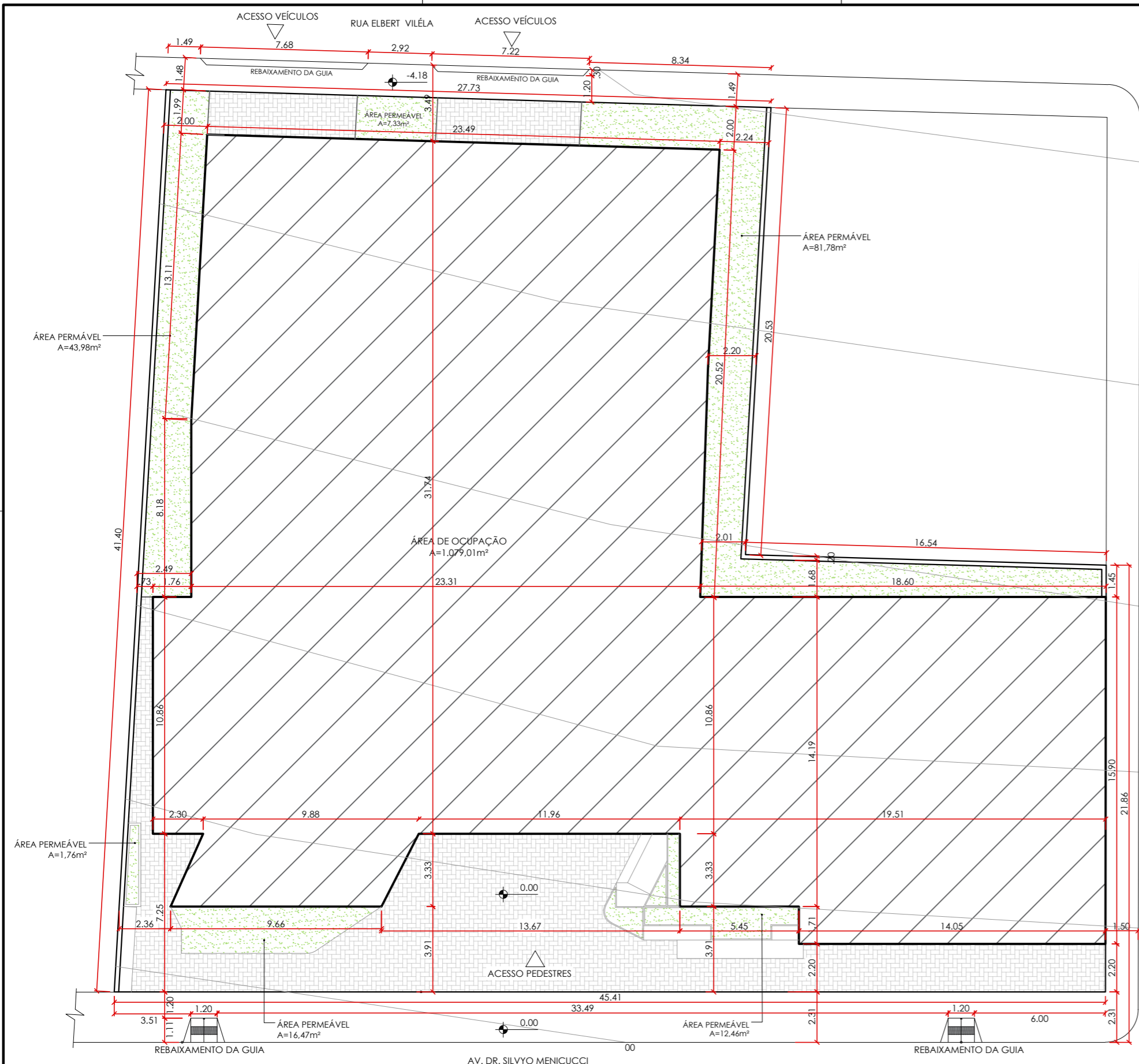
1 PLANTA DE IMPLANTAÇÃO esc 1:200
