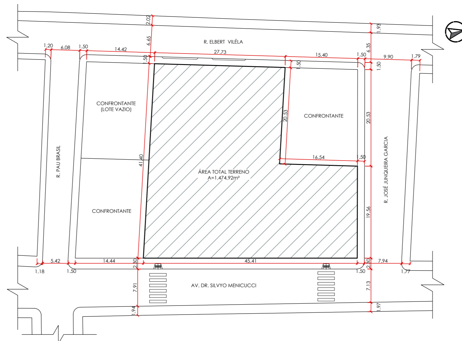
3 PLANTA DE SITUAÇÃO esc 1:500
