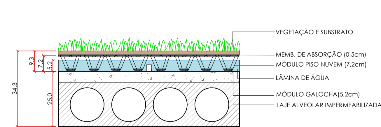
30 DET. 04 CORTE SISTEMA HIDROMODULAR esc 1:10
