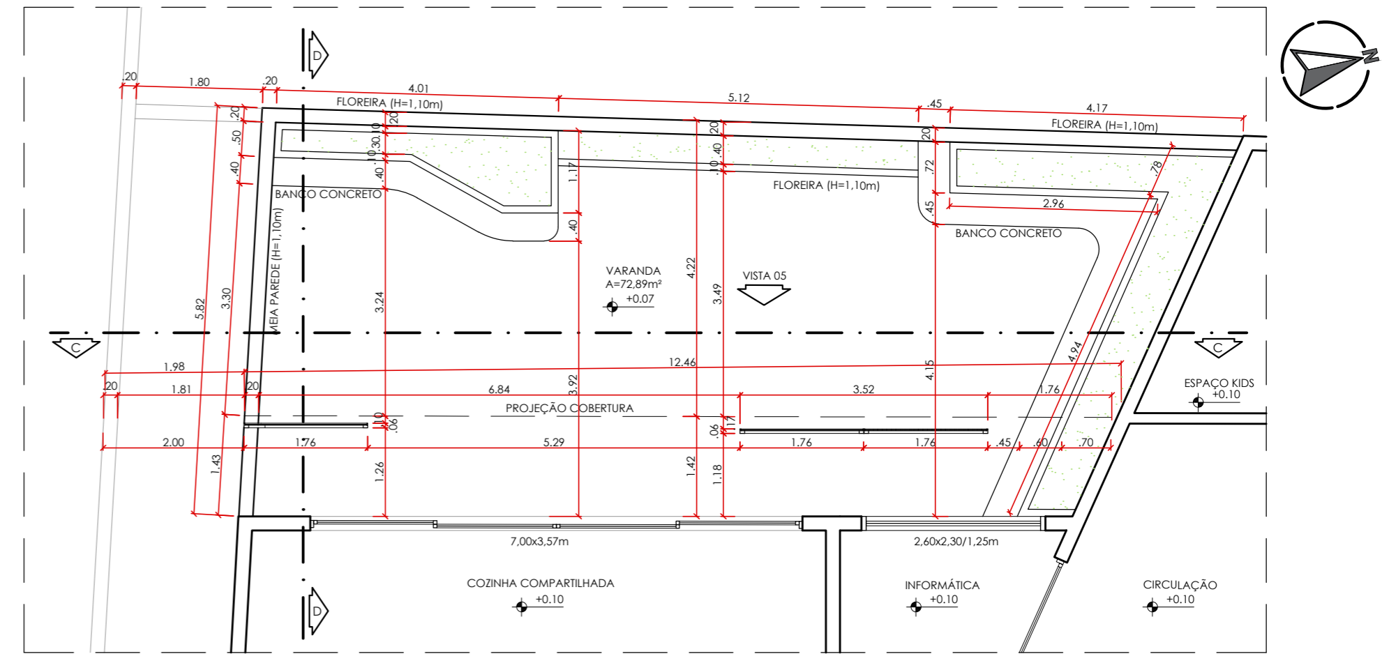
15 PLANTA BAIXA VARANDA TÉRREO esc 1:75
