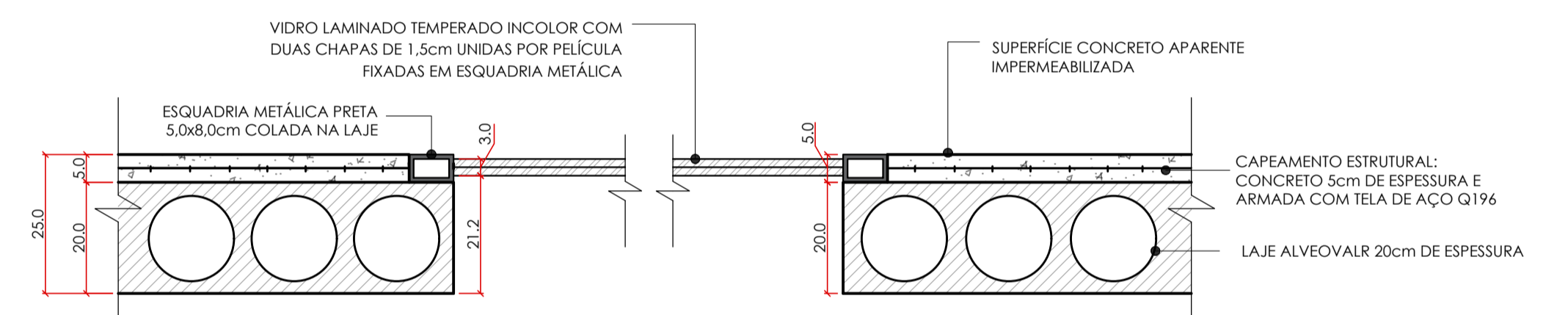
29 DET. 06 CORTE LAJE E VIDRO esc 1:10
