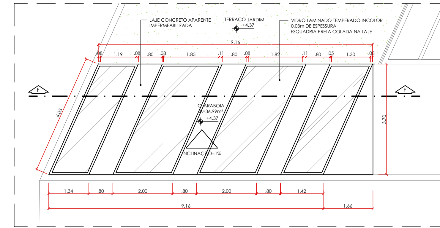
27 PLANTA CLARABOIA esc 1:75
