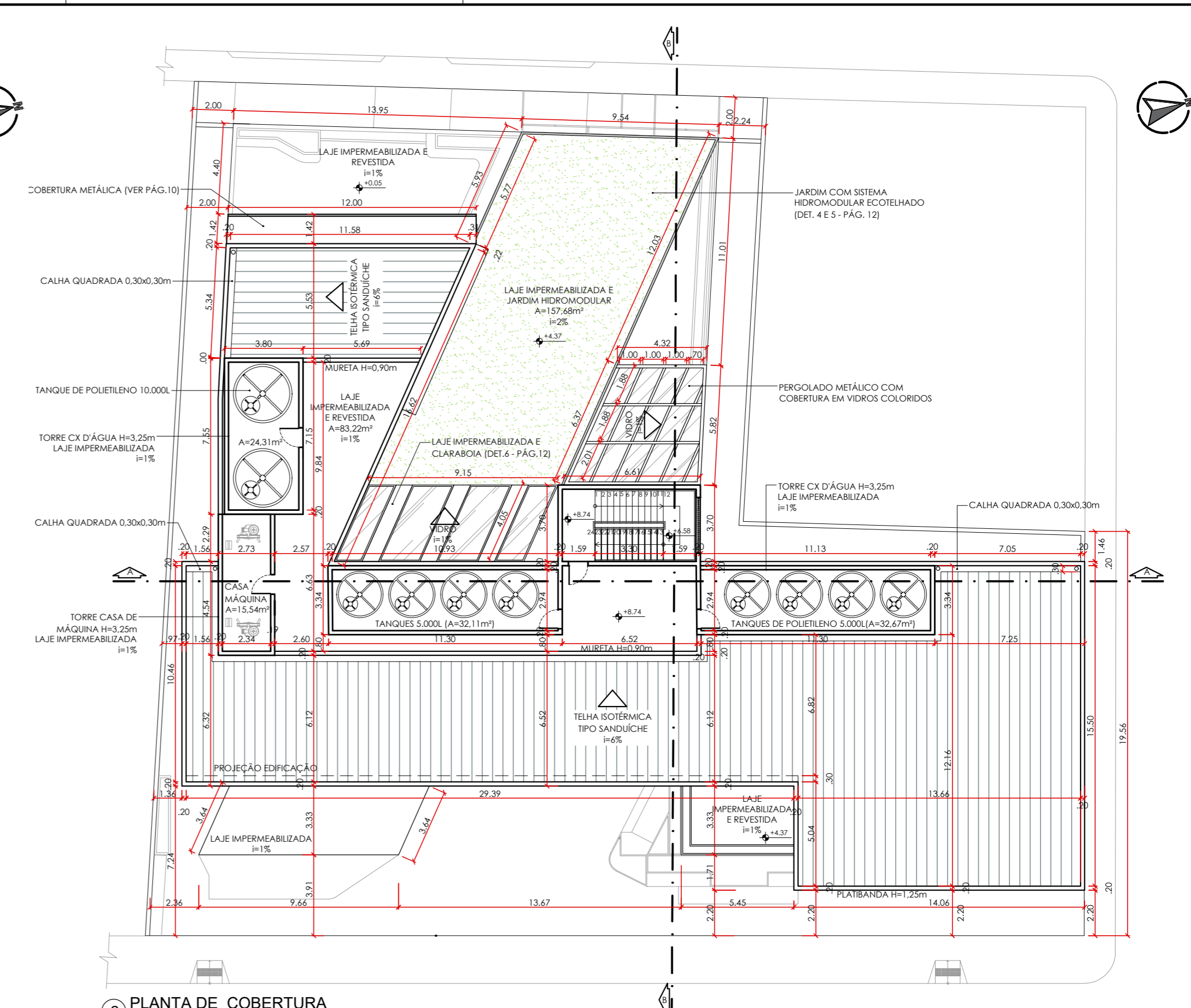
2 PLANTA DE COBERTURA esc 1:200
