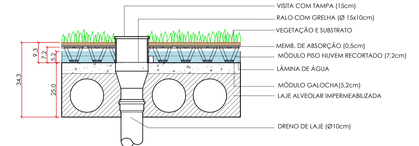
31 DET. 05 DRENAGEM DO SISTEMA esc 1:10
