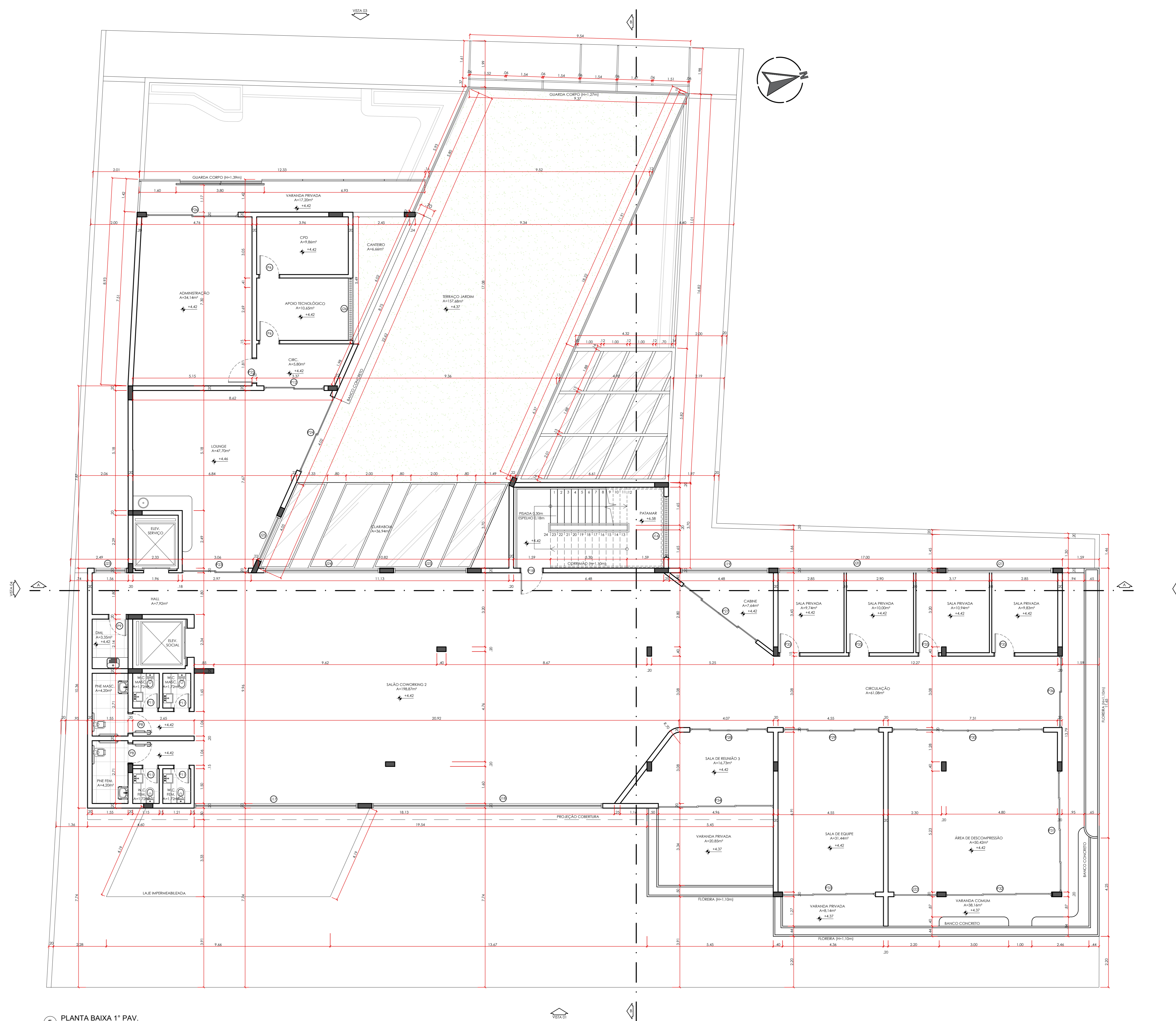
5 PLANTA BAIXA 1º PAV. 00/25,75m 466.175
