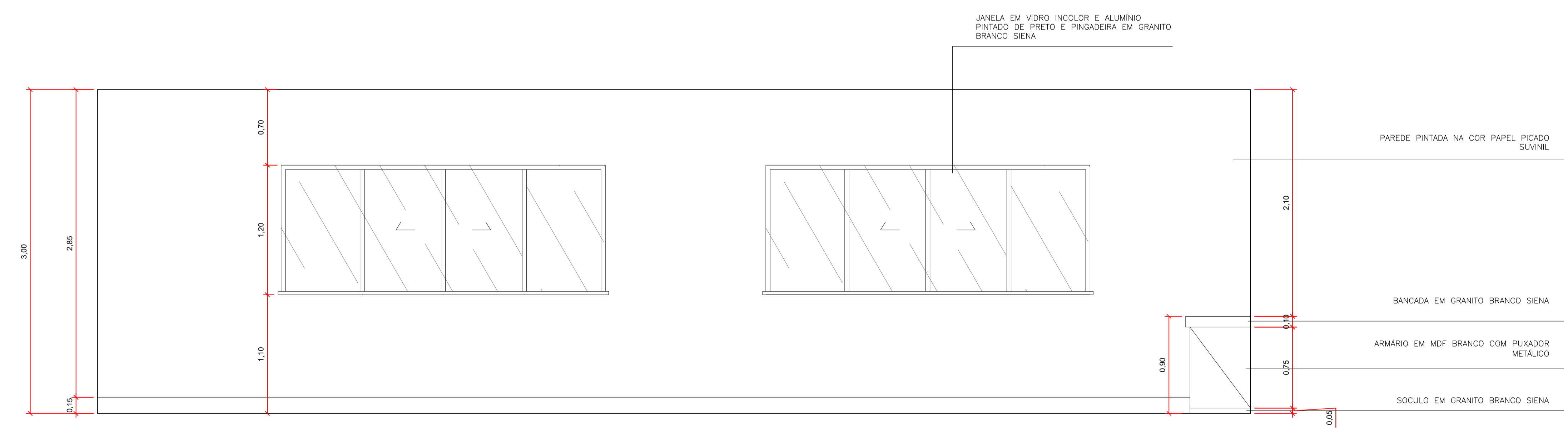
VISTA D esc 1:25
