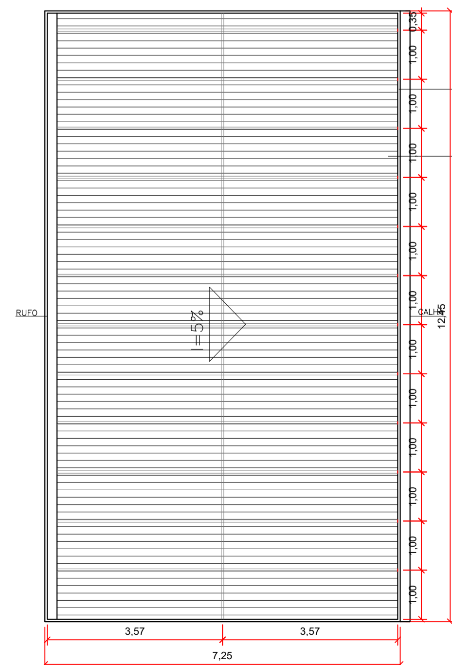
PLANTA COBERTURA POLICARBONATO esc 1:75
