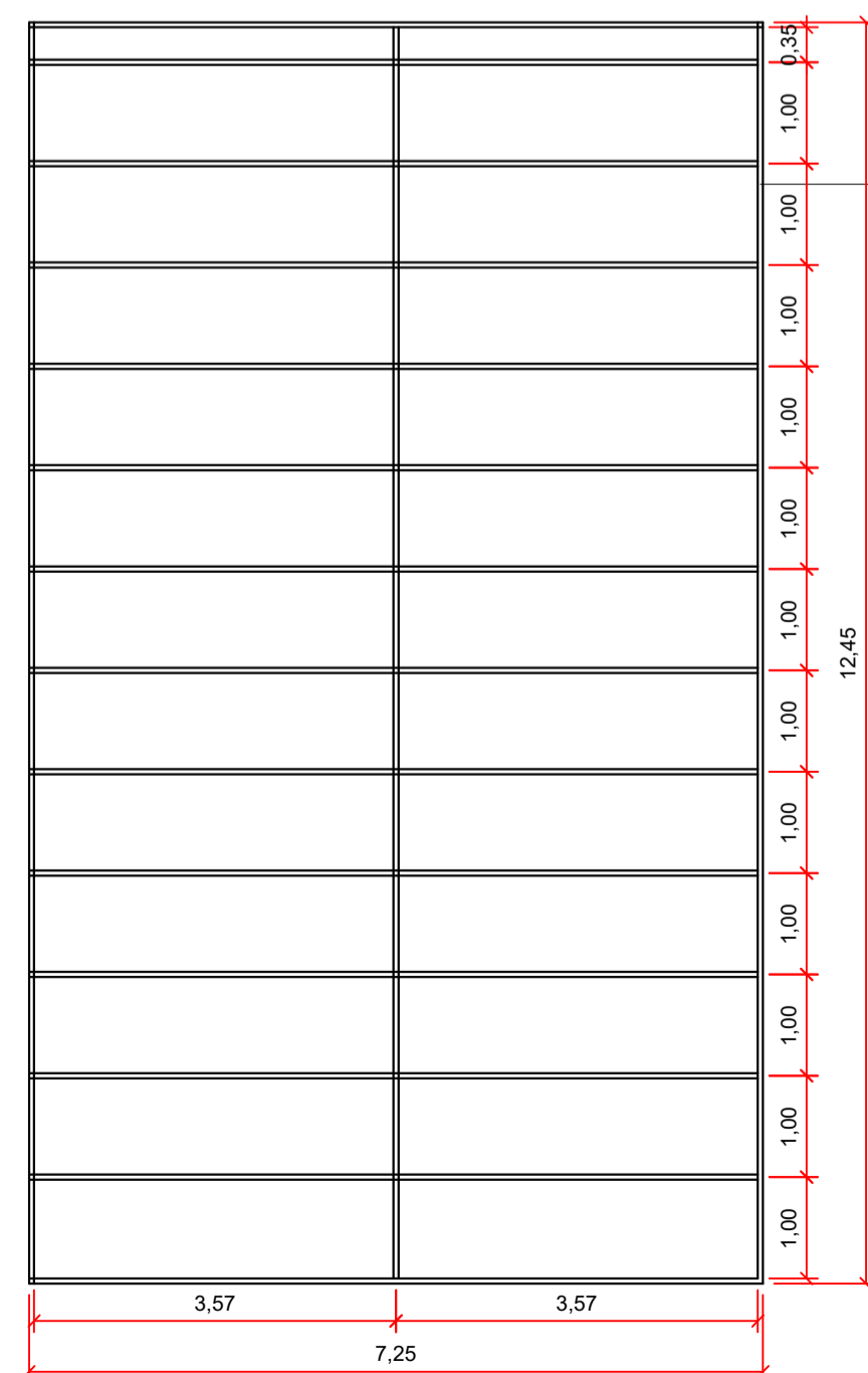
PLANTA ESTRUTURA METÁLICA esc 1:75
