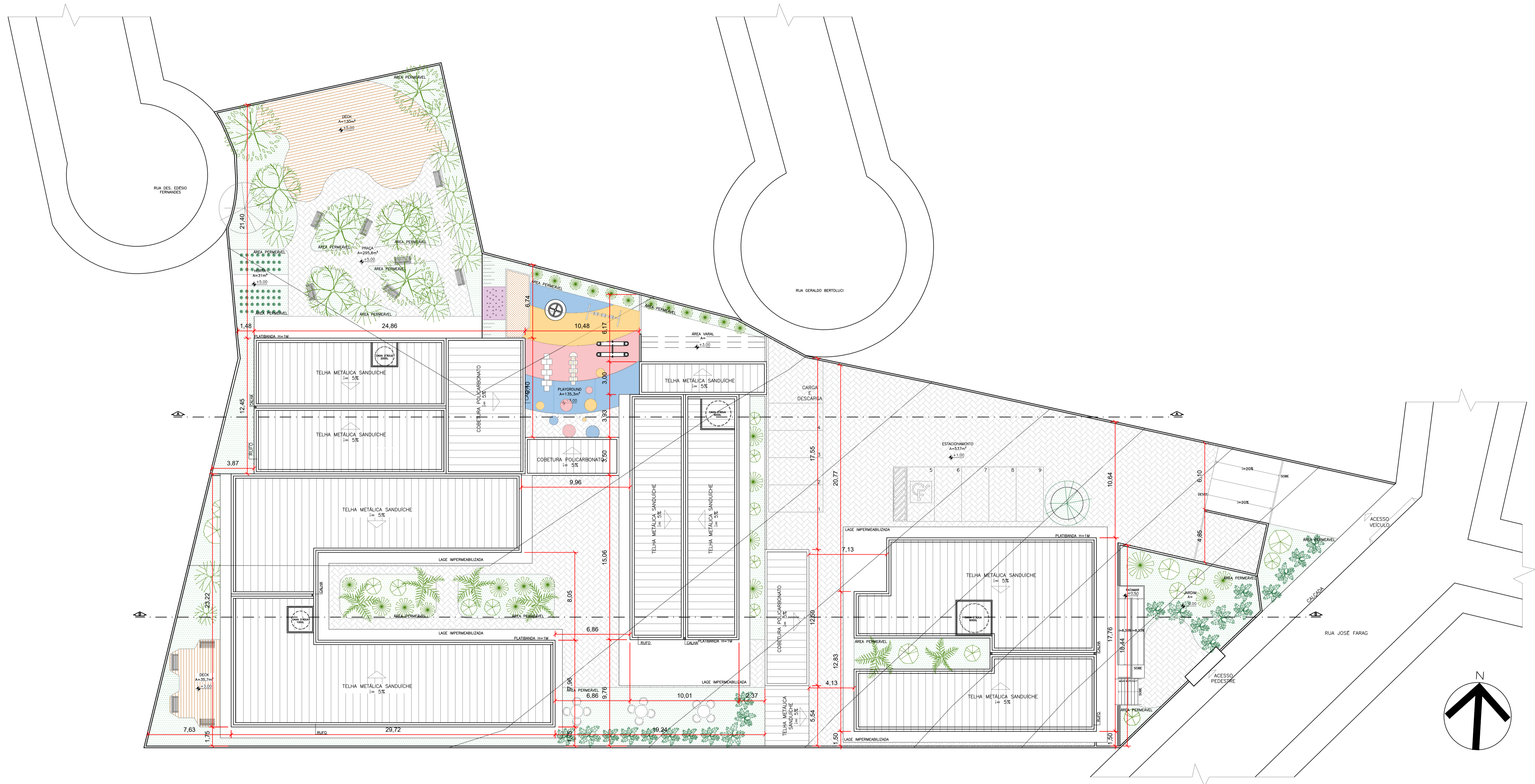
PLANTA IMPLANTAÇÃO esc 1:200
