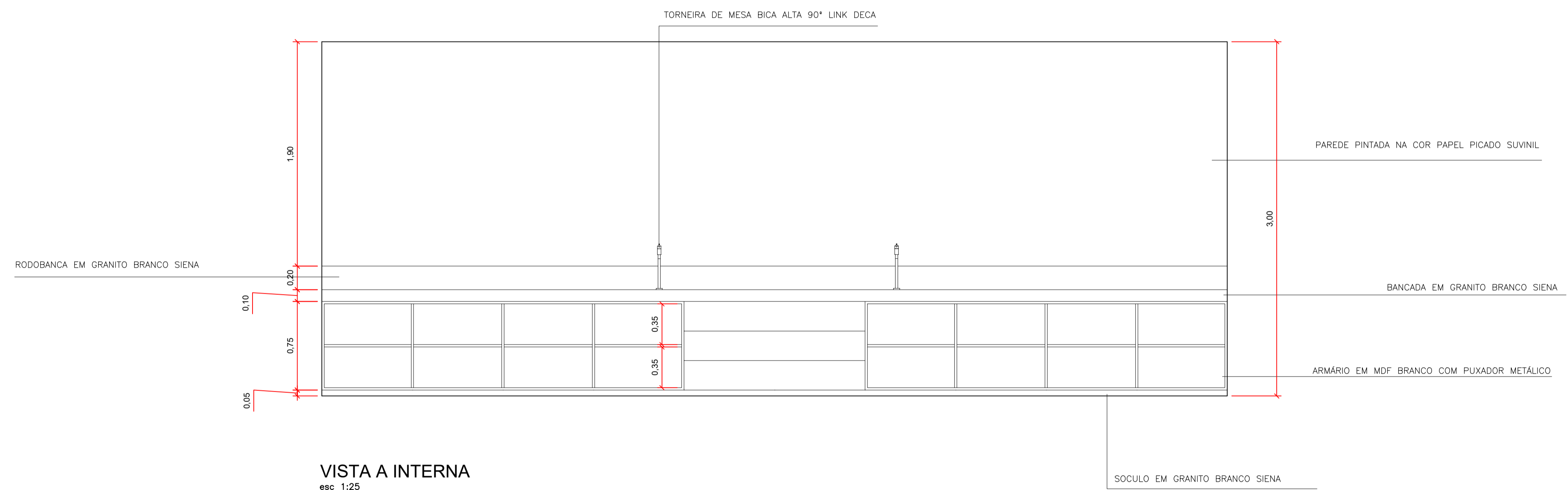
VISTA A esc 1:25
