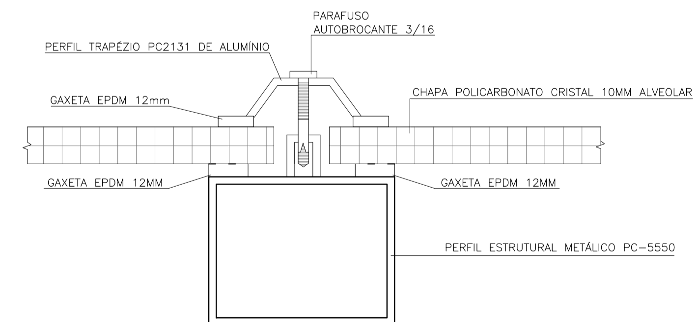
DETALHAMENTO FIXAÇÃO PLACA esc 1:1
