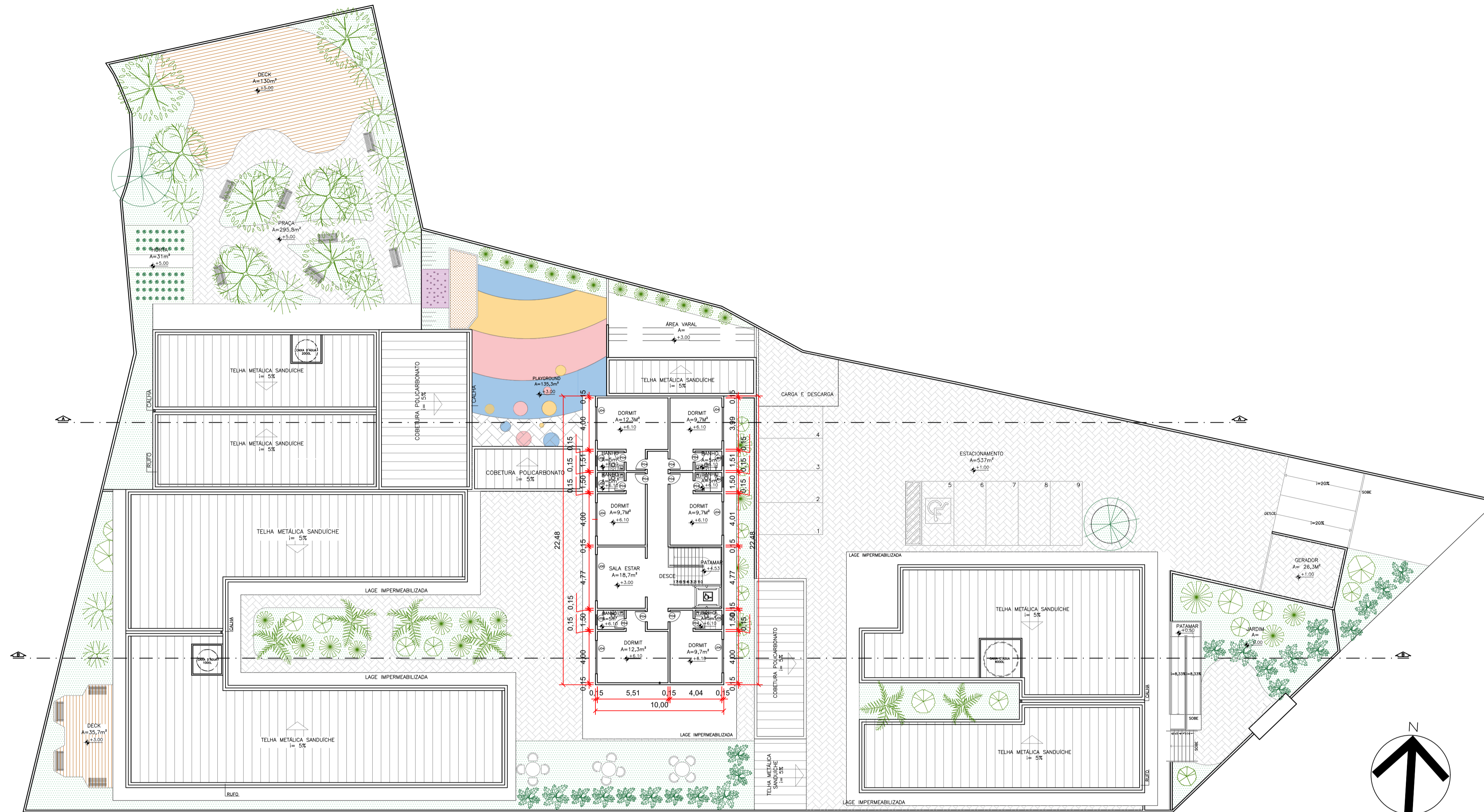
PLANTA TÉCNICA PRIMEIRO PAVIMENTO esc 1:200
