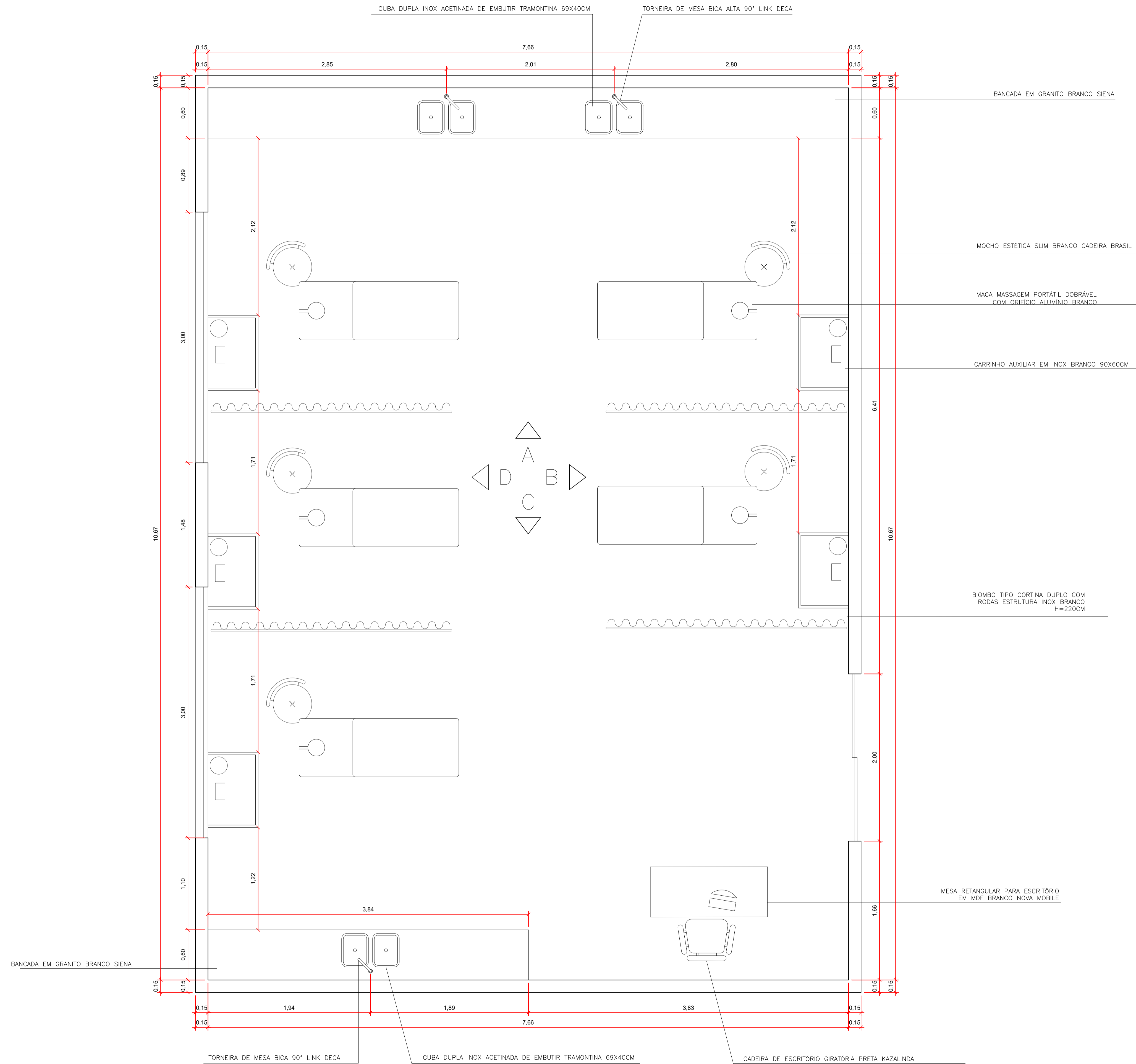
PLANTA LAYOUT esc 1:25
