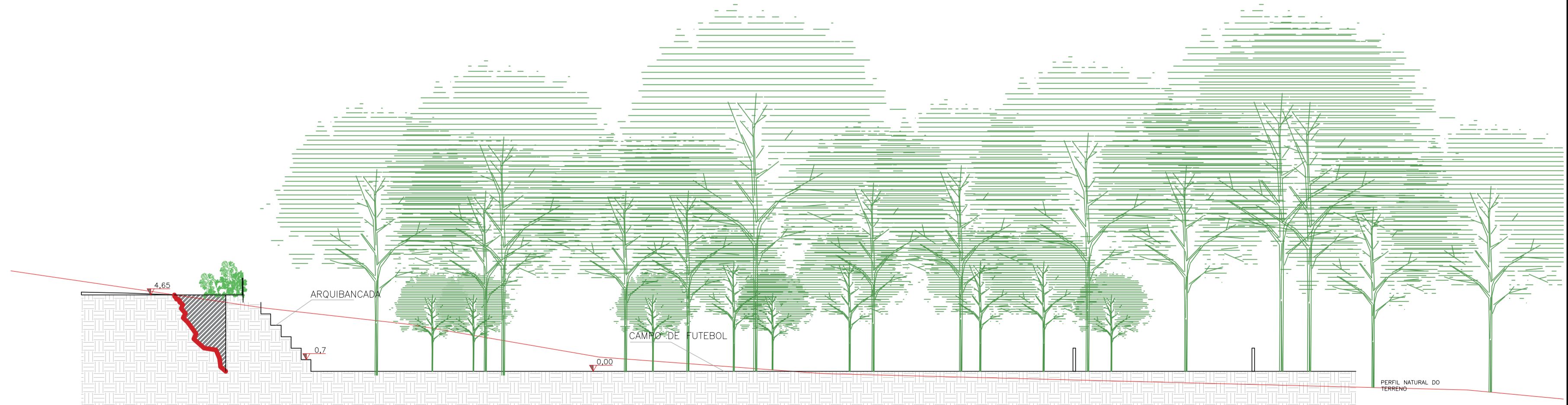
CORTE GG PRAÇA PALCO ESCALA 1:200
