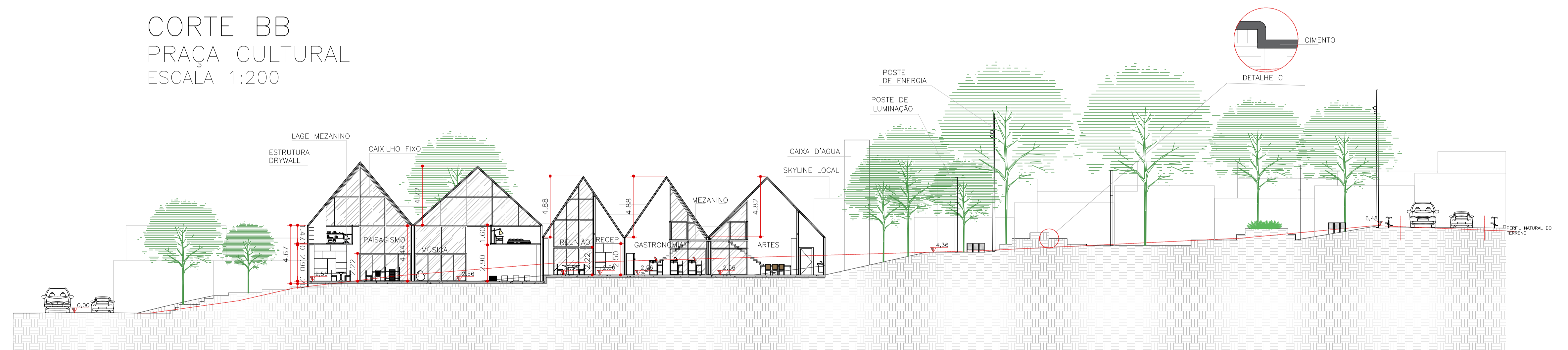
CORTE AA PRAÇA CULTURAL ESCALA 1:200
