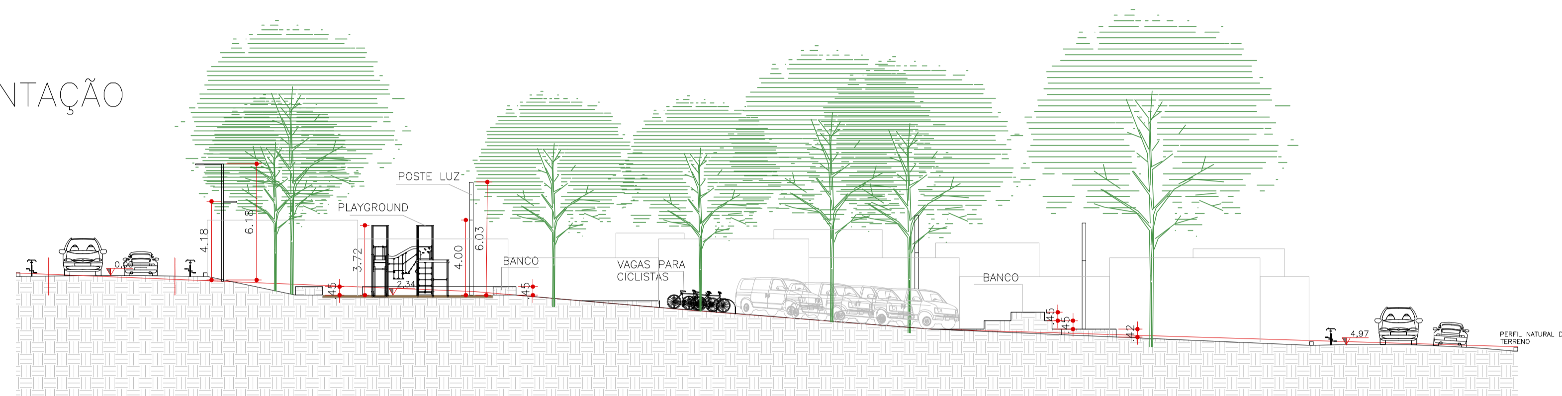
CORTE BB PRAÇA CULTURAL ESCALA 1:200
