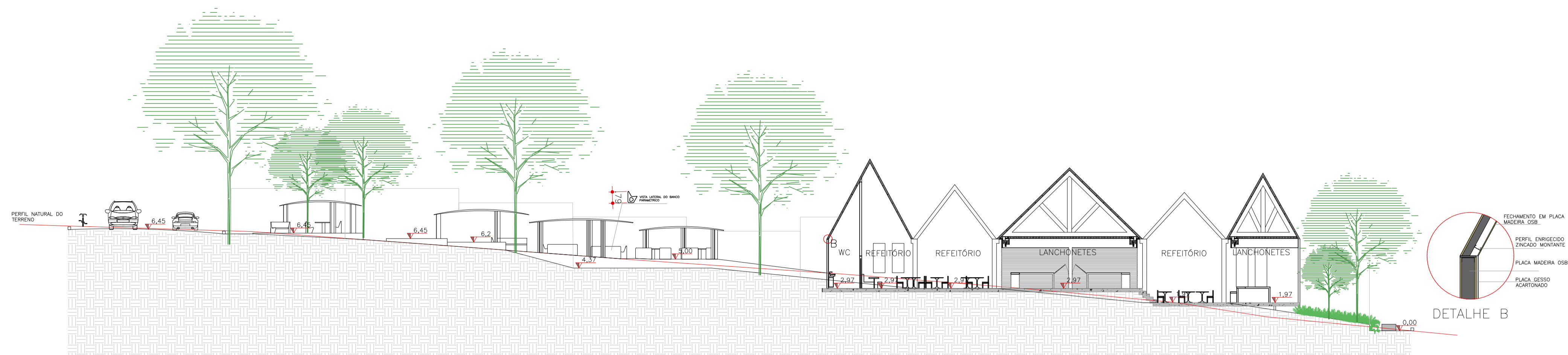
CORTE CC PRAÇA ALIMENTAÇÃO ESCALA 1:200
