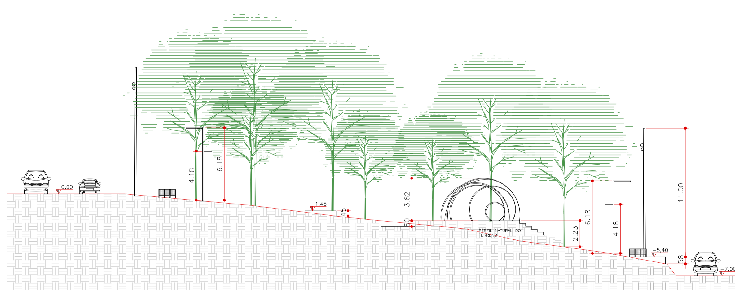
CORTE FF PRAÇA PALCO ESCALA 1:200
