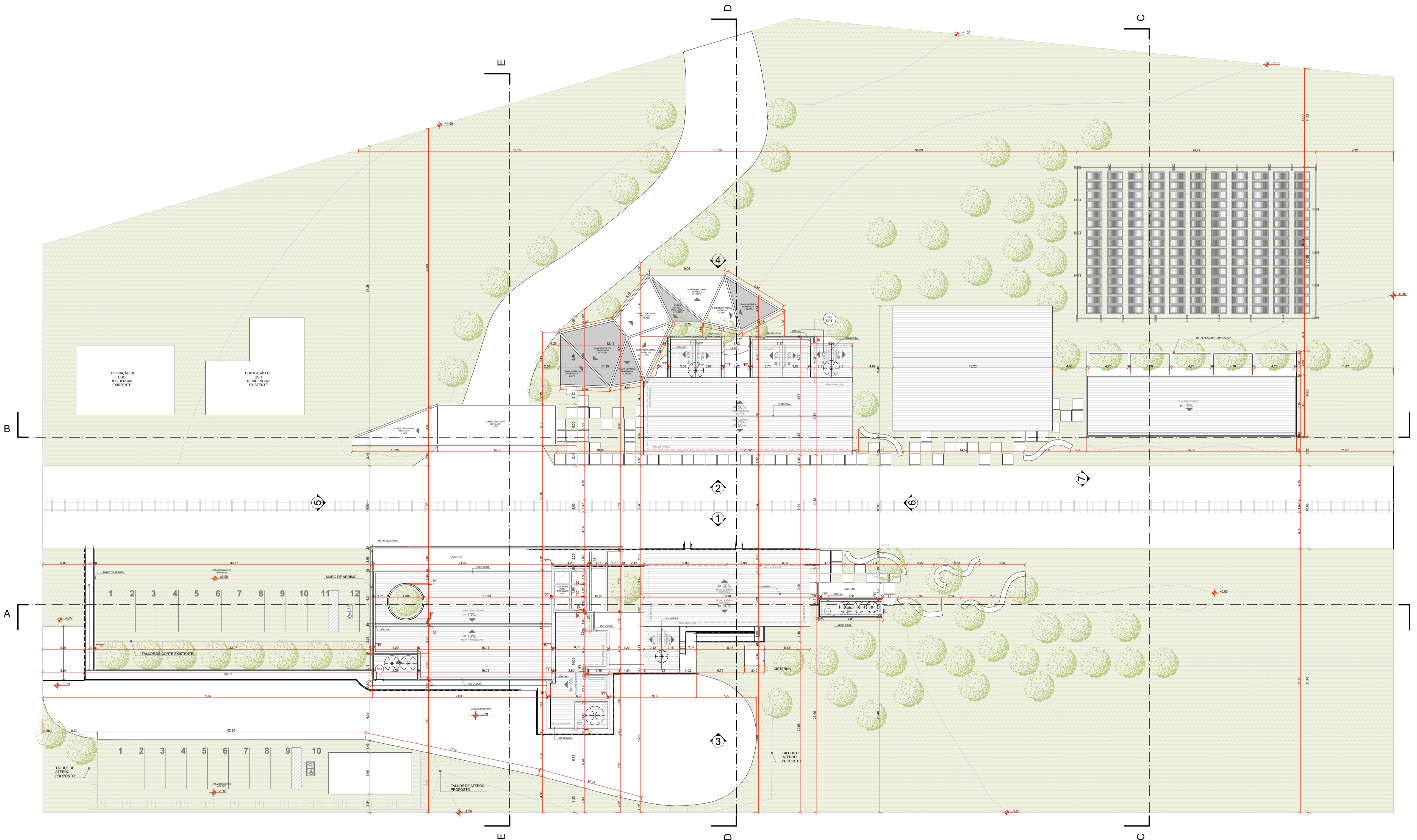
PLANTA DE IMPLANTAÇÃO E COBERTURA 1:250
