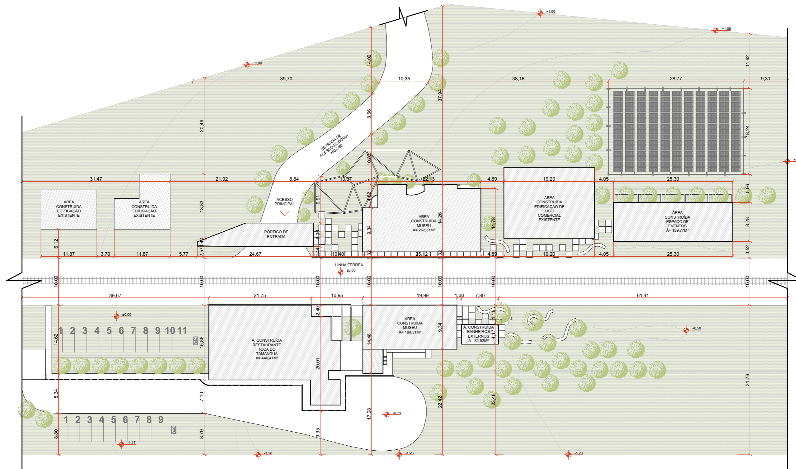
PLANTA DE SITUAÇÃO 1:500
