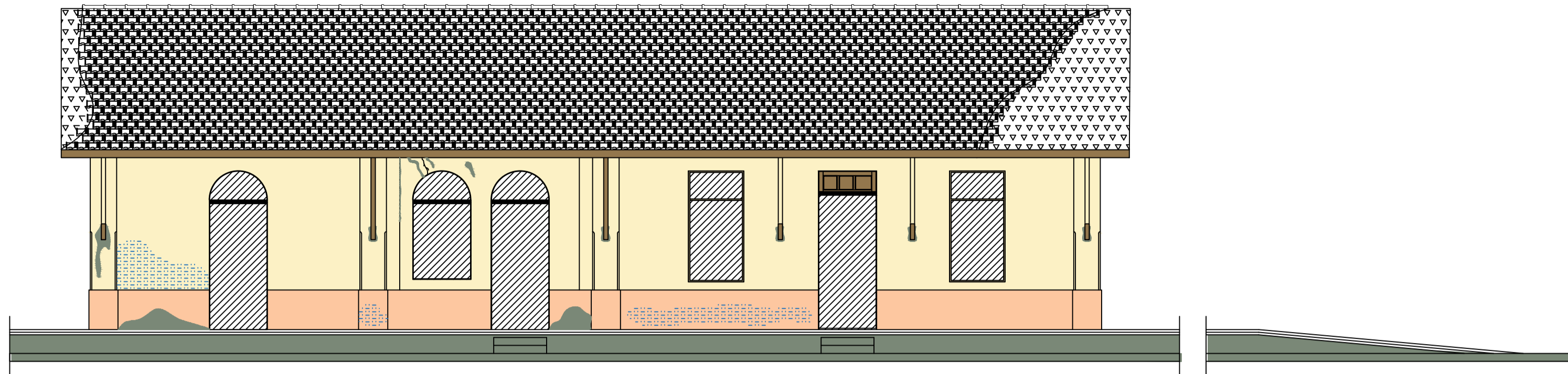
FACHADA FRONTAL ESTAÇÃO ESCALA 1/75
