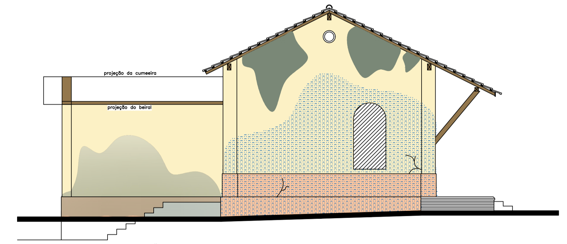
FACHADA LATERAL ESQUERDA ESTAÇÃO ESCALA 1/75
