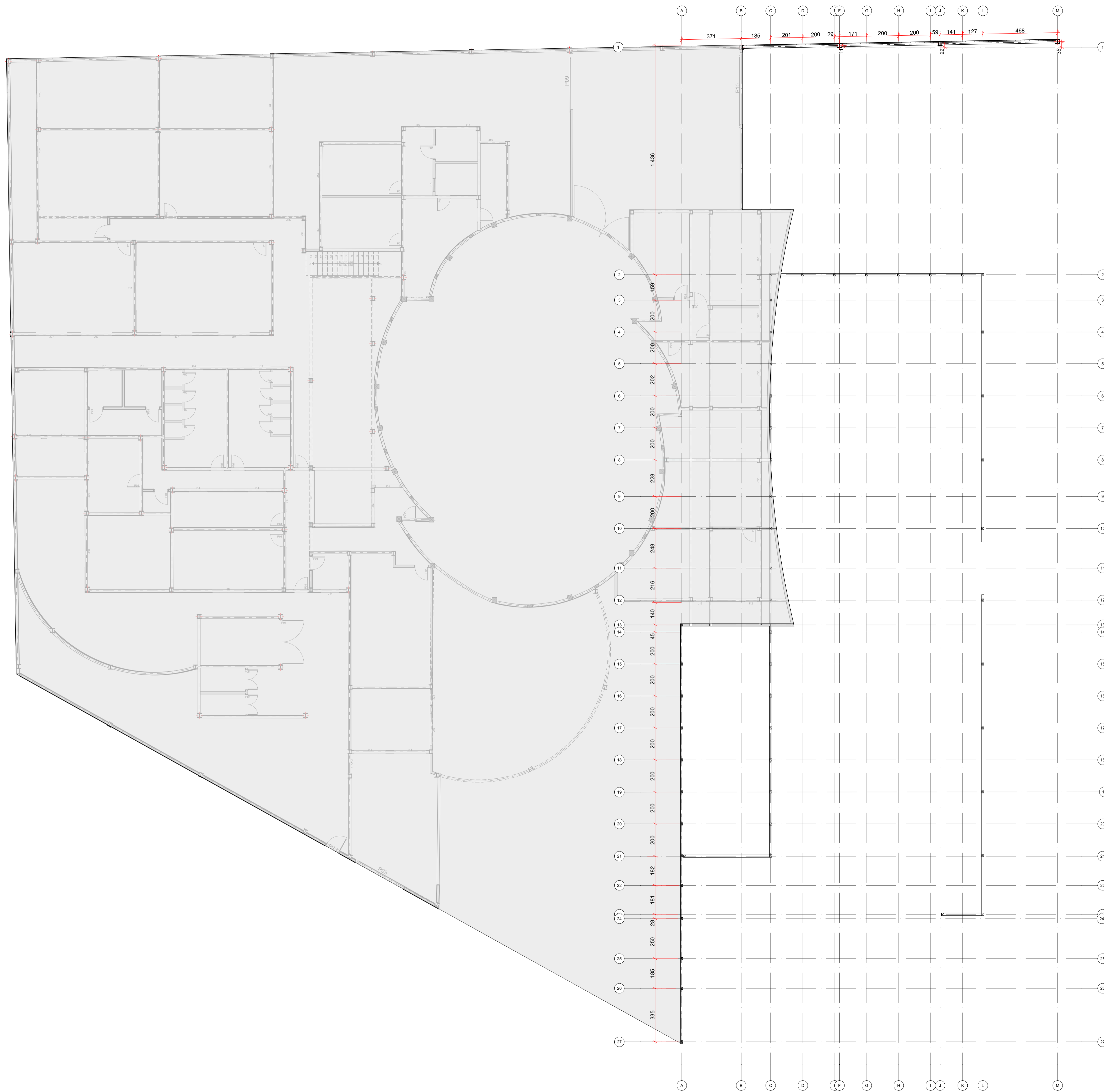
2 - Planta Estrutural Nível -3,00 - 1:125
