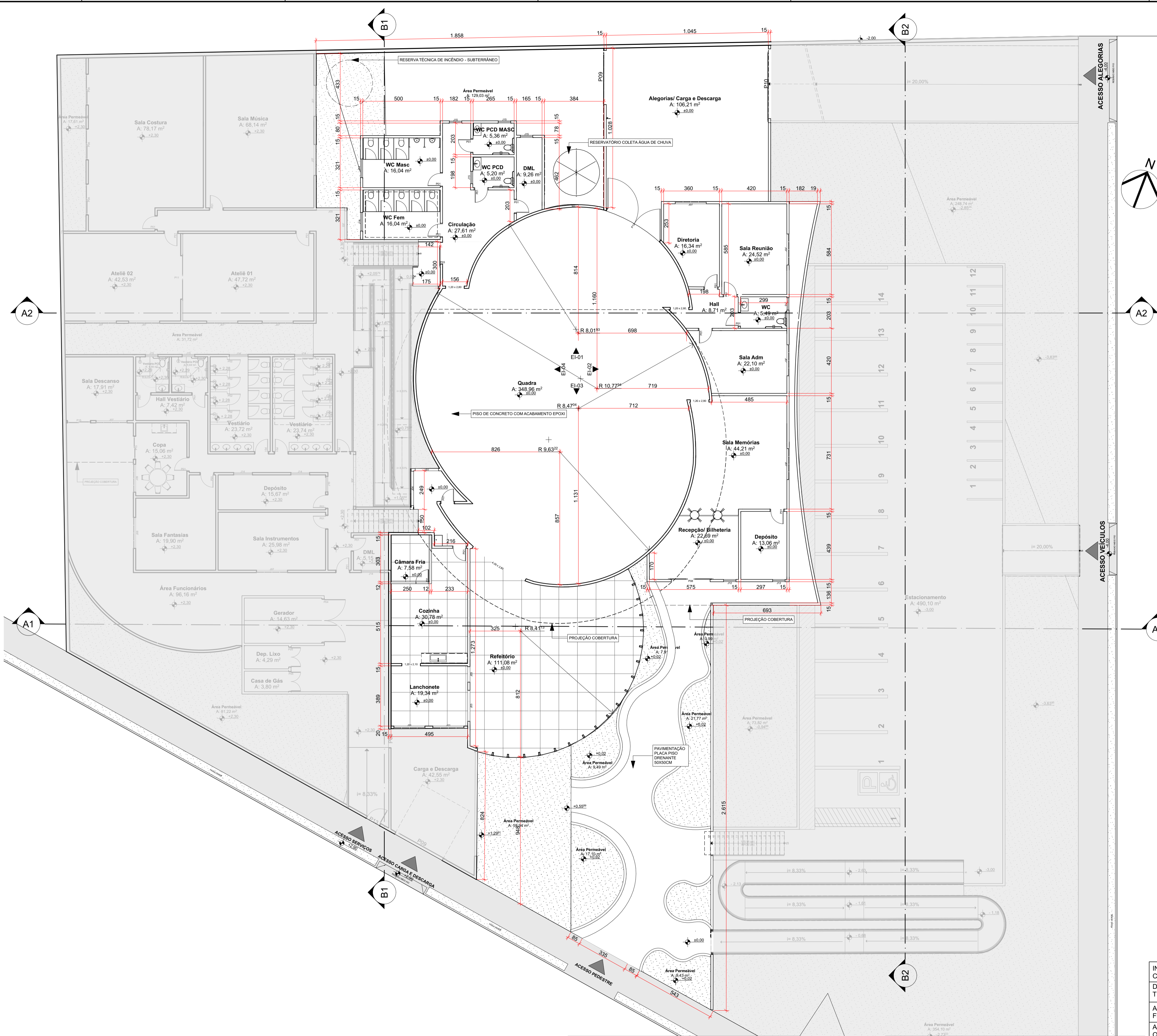
01 - Planta Baixa Nível 0 1:125
