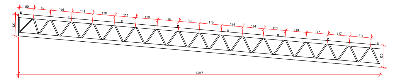
5. Elevação Trelça Metálica A 1:125
