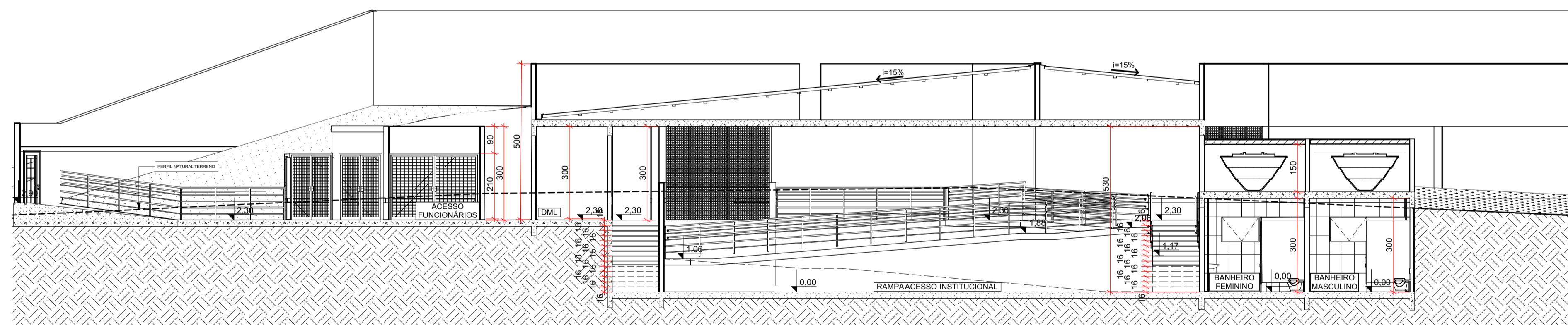
B1 - Corte 1:100
