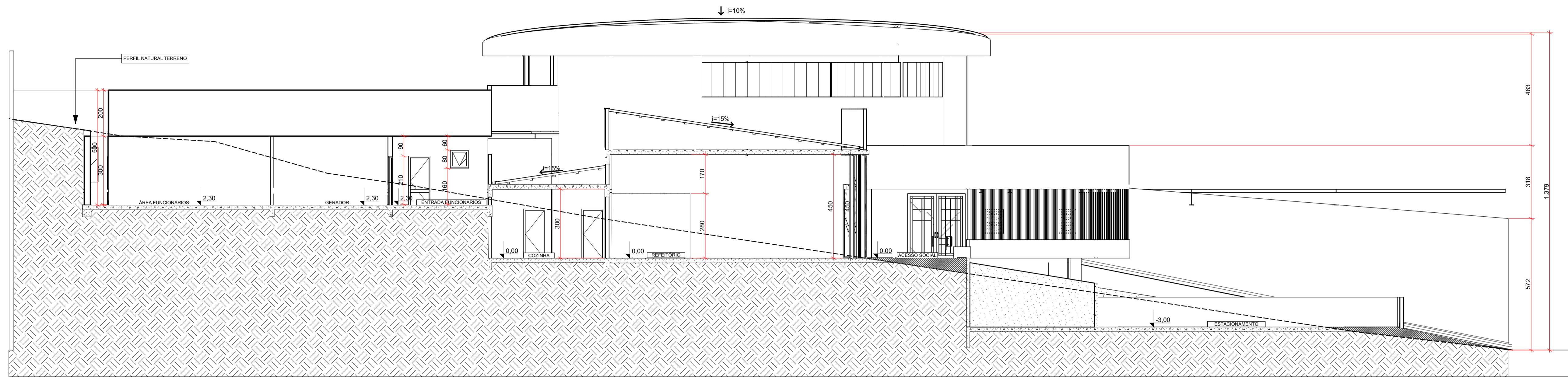
A1 - Corte 1:100
