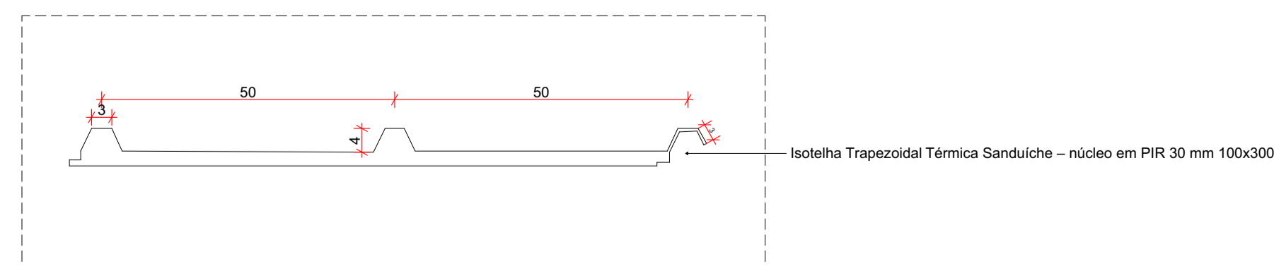
Det. 5. Det. (5) 1:5
