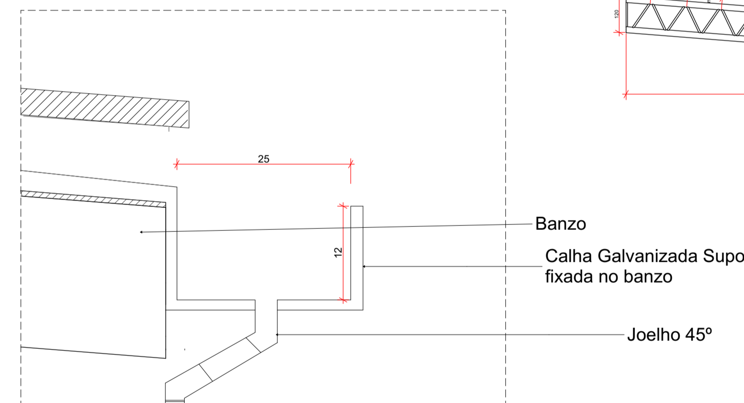
Det. 3. Det. (3) 1:5
