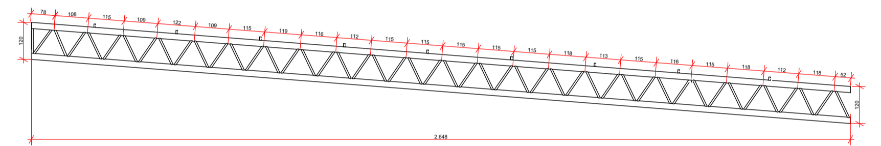
7. Elevação Trelça Metálica C 1:125
