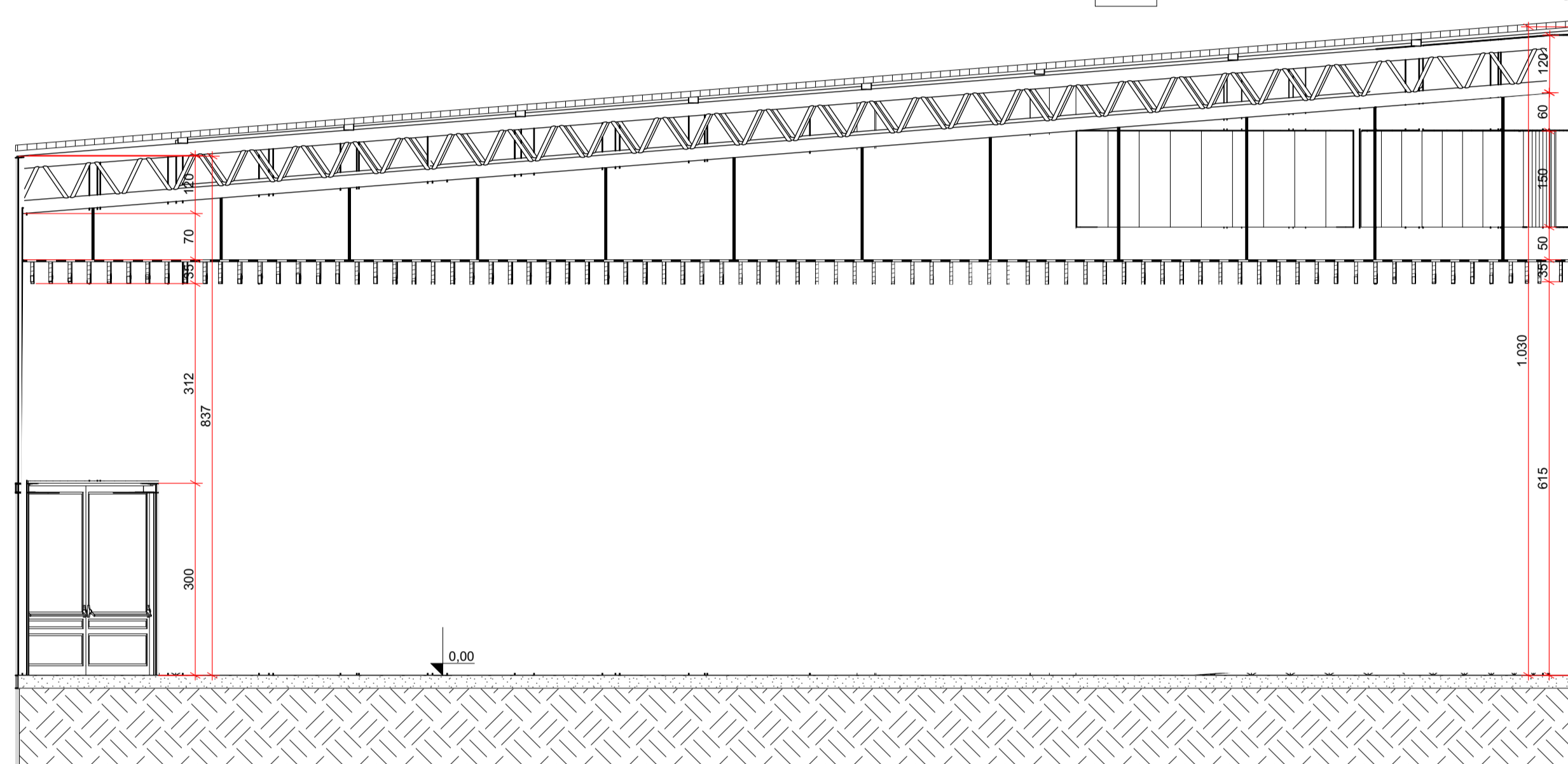
EI-02 Elevação 02 1:75
