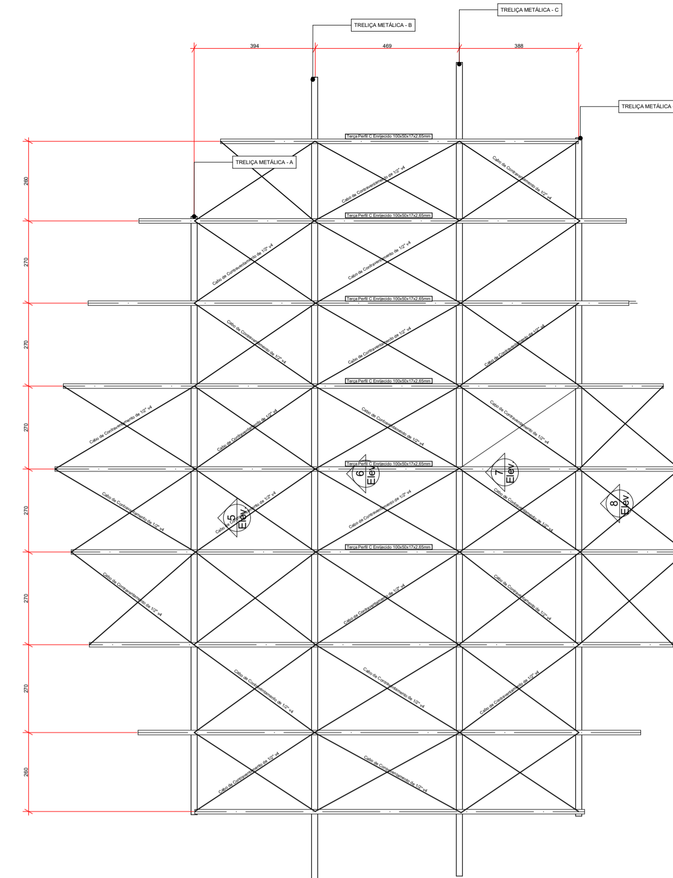
1. Detalhamento Estrutura Telhado 1:125
