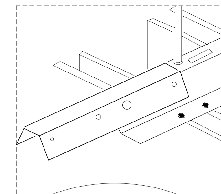
Det. 7 Det. (1)
