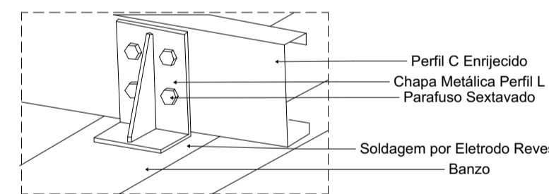
Det. 1. Det. (1) 1:5
