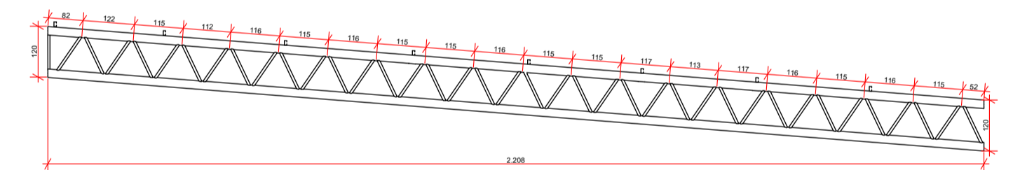
8. Elevação Trelça Metálica D 1:125
