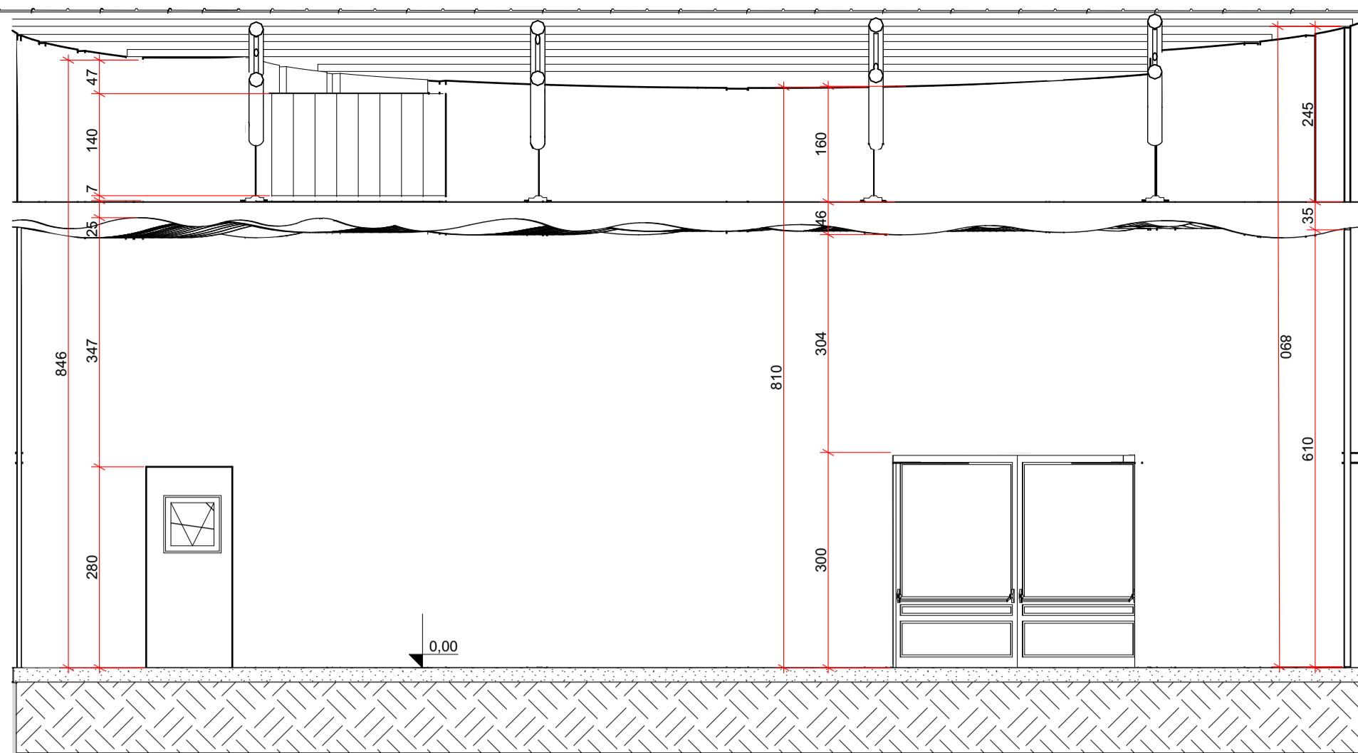
EI-01 Elevação 01 1:75
