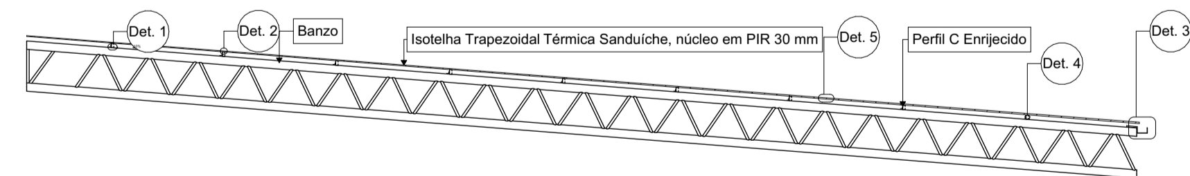
1. Detalhamento Trelça 1:125
