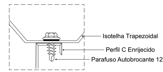
Det. 2. Det. (2) 1:5
