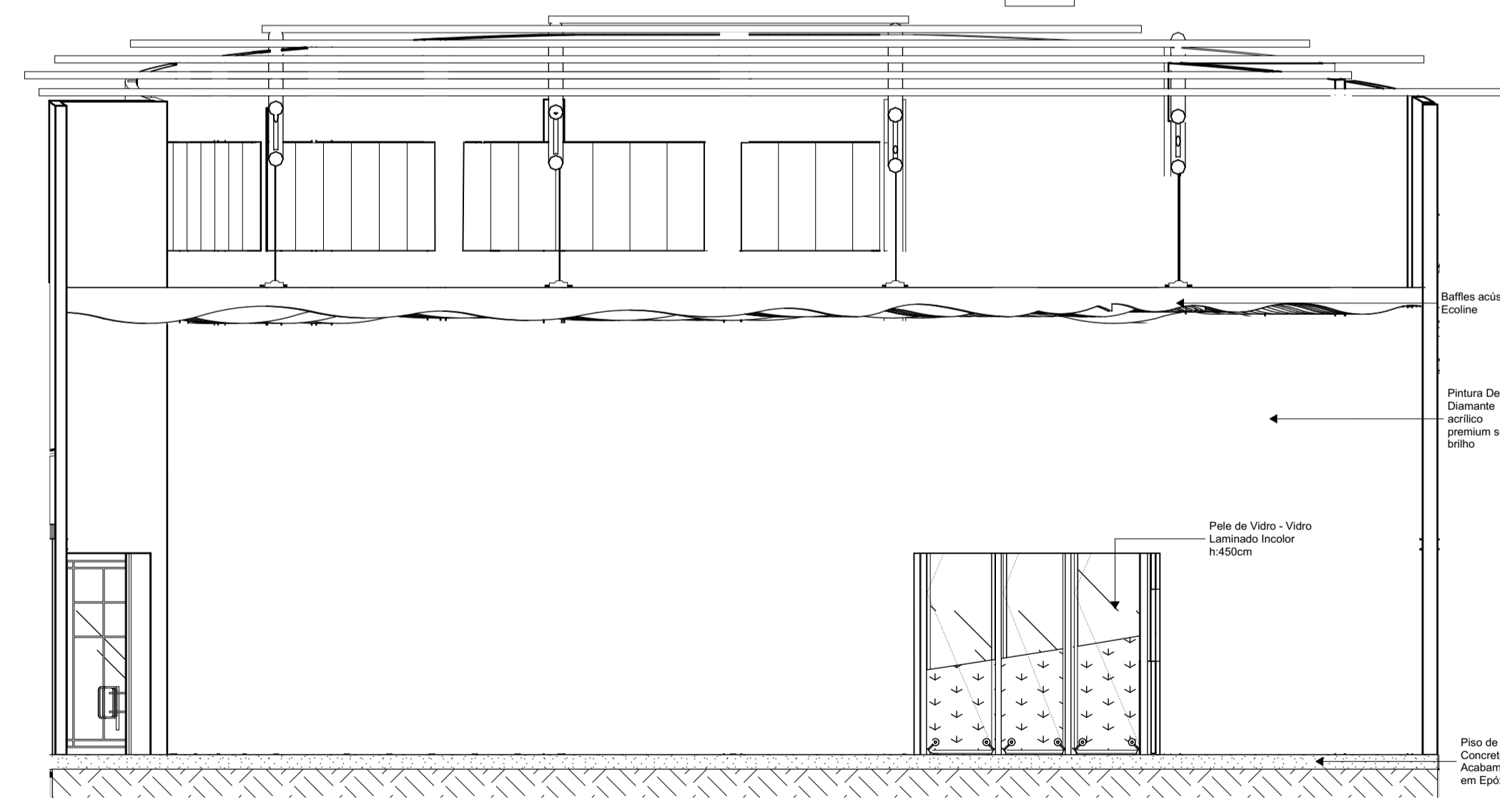
EI-03 03 1:75
