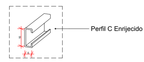
Det. 4. Det. (4) 1:5
