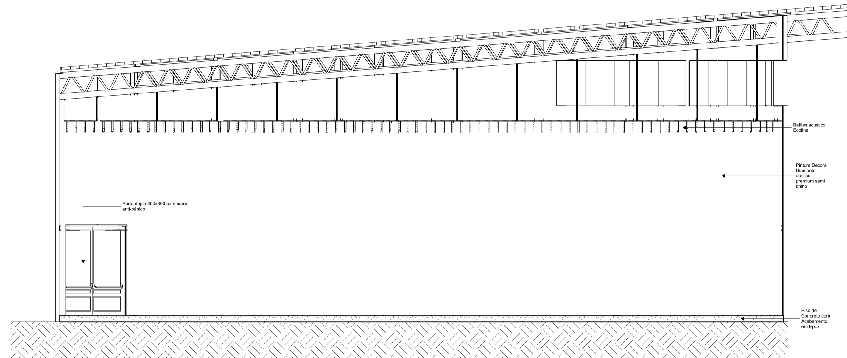
EI-02 02 (1) 1:75
