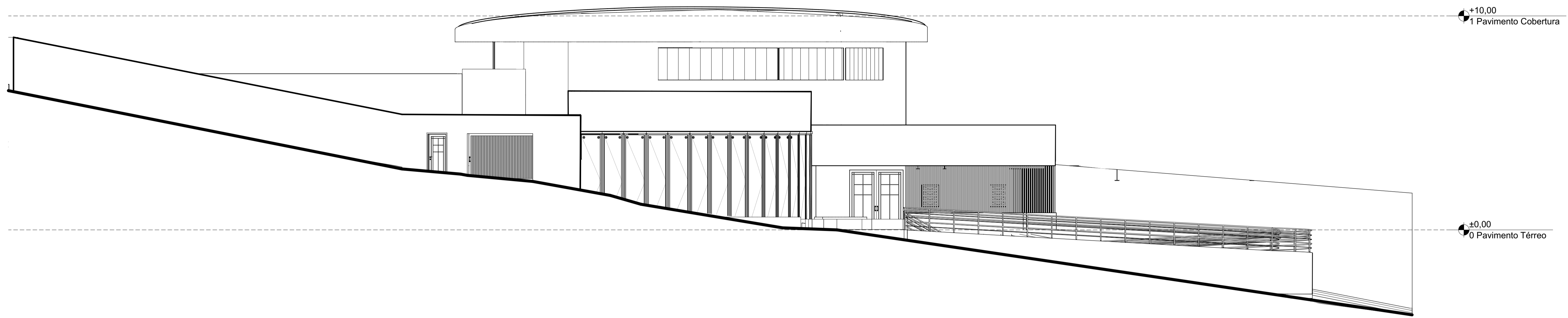
1 Fachada Frontal 1:100
