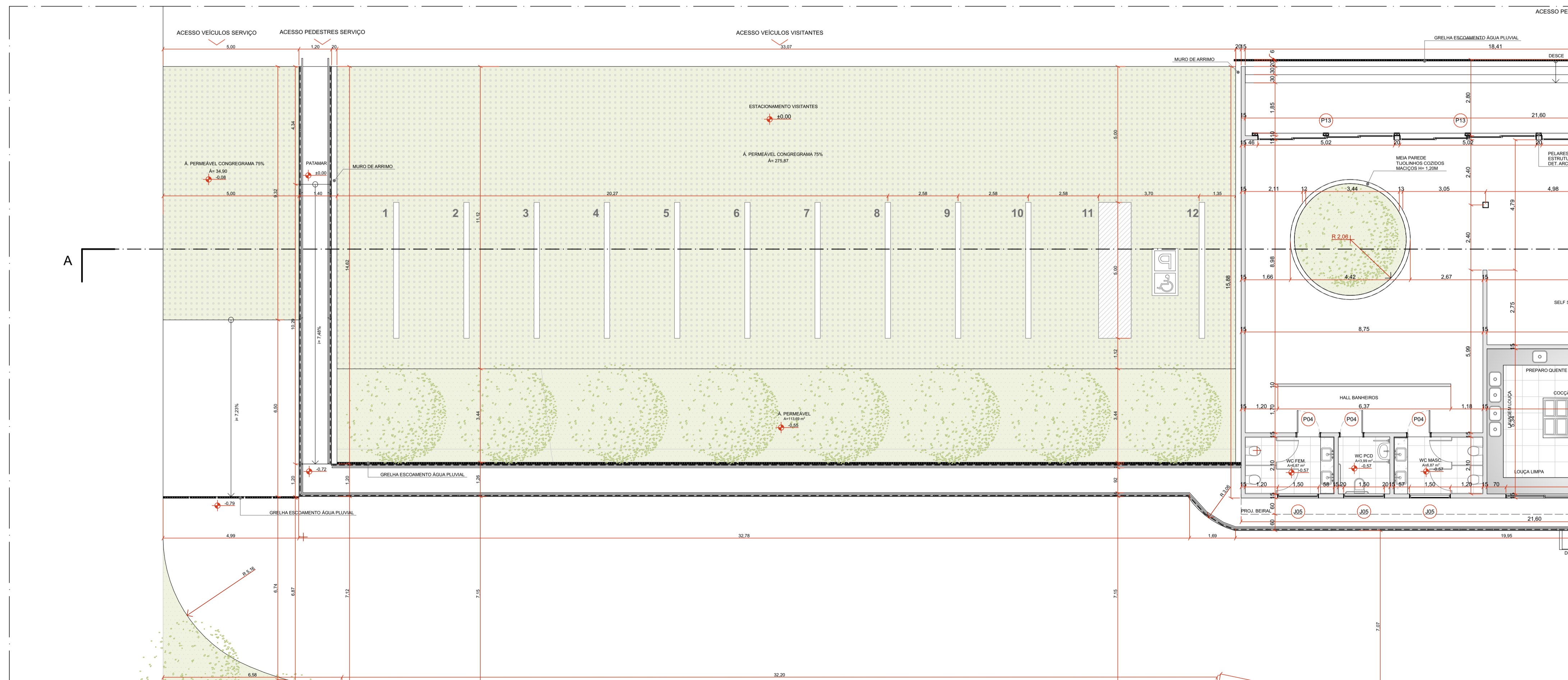
PLANTA TÉCNICA ESTACIONAMENTO VISITANTES 1:100
