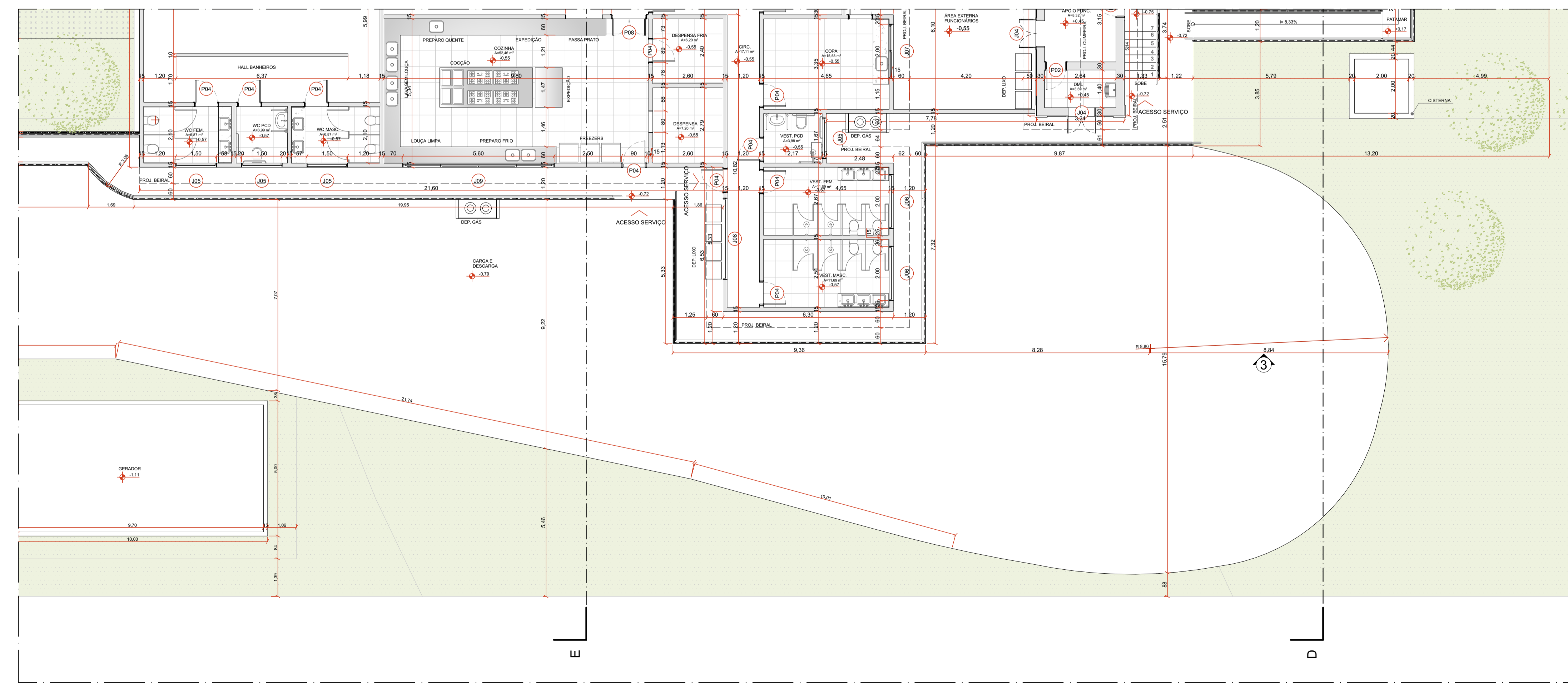
PLANTA TÉCNICA CARGA E DESCARGA 1:100
