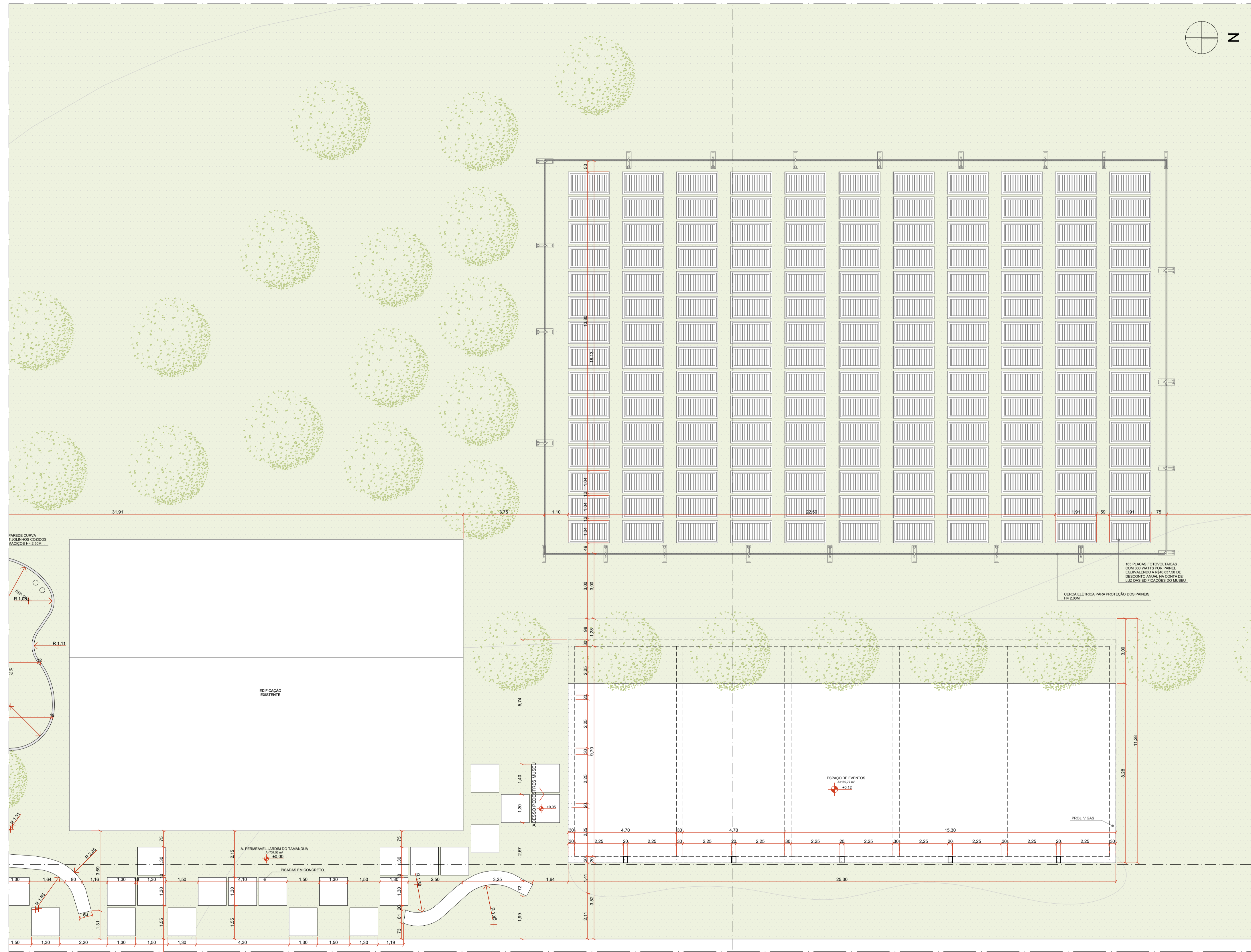
PLANTA TÉCNICA ESPAÇO DE EVENTOS 1:100
