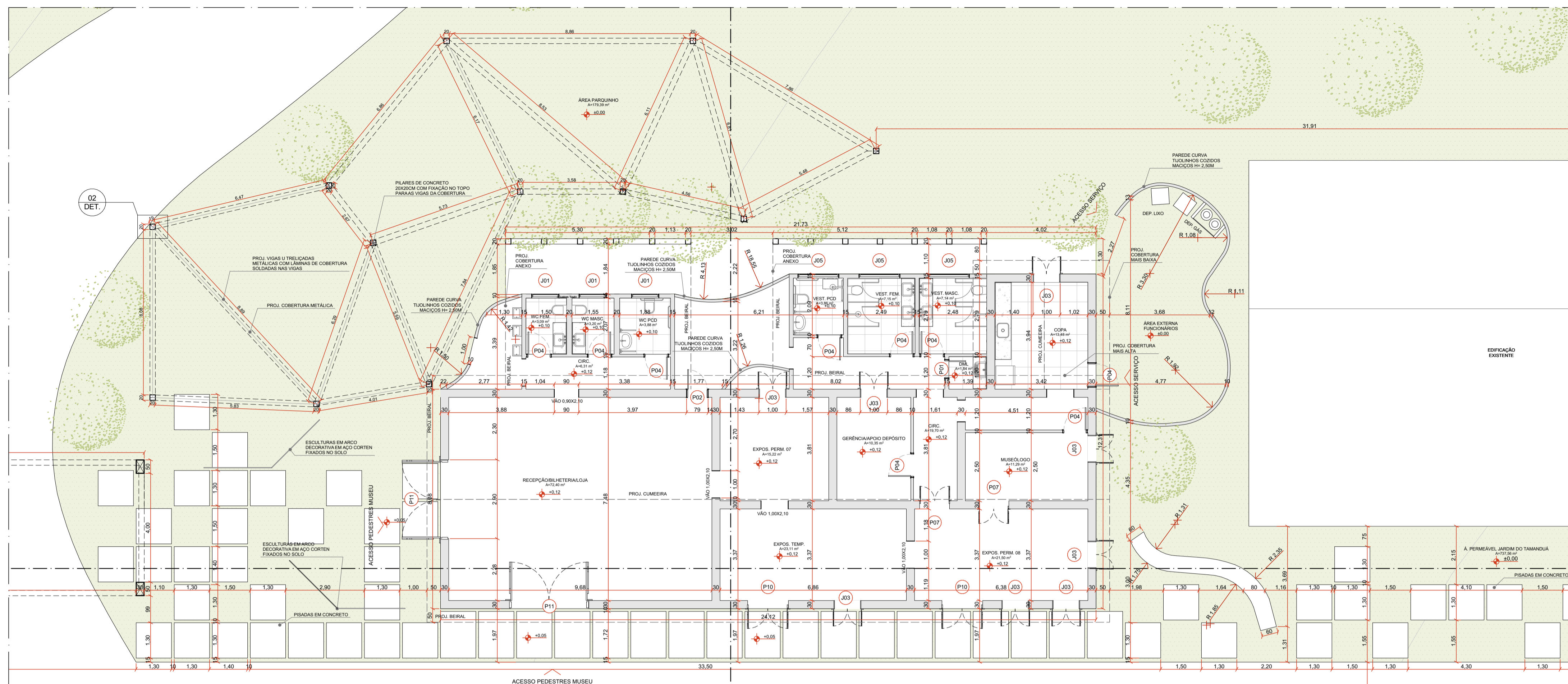
PLANTA TÉCNICA ARMAZÉM 1:100
