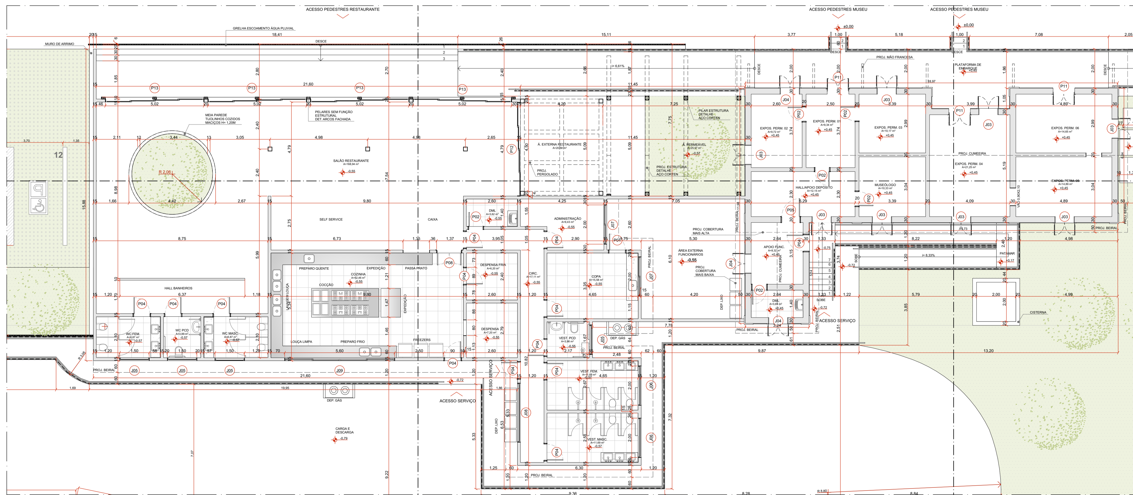
PLANTA TÉCNICA RESTAURANTE E ESTAÇÃO 1:100
